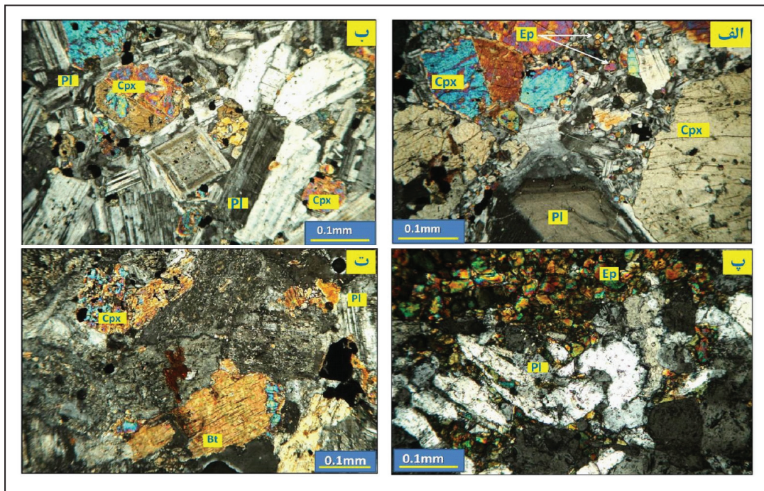
شکل ۴- تصویر میکروسکوپی سنگ‌های درونگیر و میزبان کانه‌زایی آهن در کانسار کوه بابا. الف) واحد گابرو نوریت با بافت گرانولار که حاوی کانی‌های پیروکسن و پلاژیوکلاز است؛ ب) توده نفوذی گابرو نوریت با بافت ساب‌افیتییک؛ پ) دگرسانی اپیدوتی در واحد دیوریت؛ ت) واحد بیوتیت گابرو با بافت هیپیدومورف گرانولار (پلاژیوکلاز= Pl، کلینوپيروكسن= Cpx، اپیدوت= Ep، بیوتیت= Bt) (نور تصاویر: XPL).
