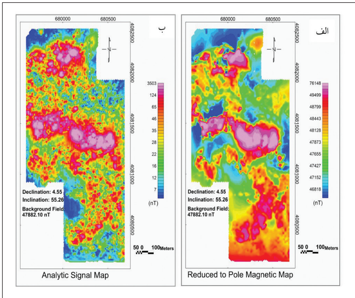
شکل ۹-الف) نقشه برگردان به قطب؛ ب) نقشه سیگنال تحلیلی کانسار آهن کوه بابا که نشان‌دهنده ابعاد ناهنجاری شمالی (۳۰۰ × ۲۰۰) و مرکزی (۵۵۰ × ۱۷۰) است.
