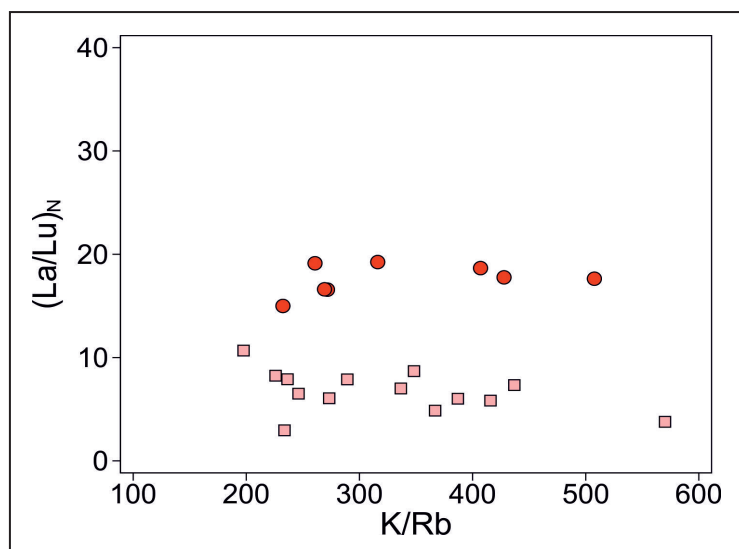
شکل ۴- الف) جانمایی لوکوگرانیت‌ها بر روی نمودار (\text{LREE}/\text{HREE})_N در برابر \text{K}/\text{Rb} به عنوان شاخص تفریق. به دو روند جداگانه آن‌ها توجه نمایید. علائم مانند شکل ۲.
