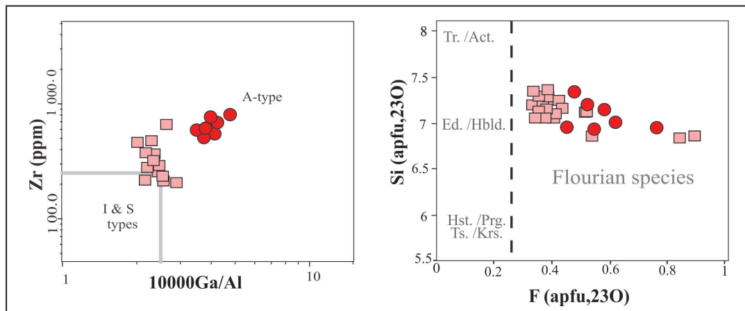
شکل ۳- الف) ترکیب آمفیبول‌های کلسیک لوکوگرانیت‌ها در نمودار سیلیس در برابر محتوای فلوتور. Hst = هاستینگزیت، Prg = پارگازیت، Tr = چرماکیت، Krs = کرسوتیت، Ed = ادنیت، Hbld = هورنبلند، Act = اکتینولیت، Tr = ترمولیت؛ (ب) جانمایی نمونه‌ها بر روی نمودار تفکیکی Whalen et al. (1987) (علامه مانند شکل ۲).
