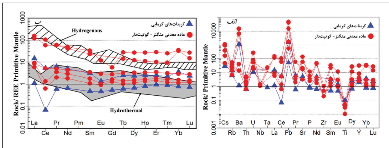
شکل ۹- الگوی بهنجار شده عناصر جزئی و خاکی کمیاب در نمونه‌های منگنز-گوتیت دار و کربنات‌های گرمایی، الف) نمودار عناصر جزئی بهنجار شده نسبت به گوشته اولیه (McDonough and Sun, 1995) در کانسار حلب، ب) نمودار عناصر خاکی کمیاب بهنجار شده نسبت به گوشته اولیه (McDonough and Sun, 1995) در کانسار حلب و مقایسه الگوی توزیع عناصر خاکی کمیاب کانسنگ منگنز حلب با کانسارهای گرمایی (Toth, 1980) و آب‌زاد.
