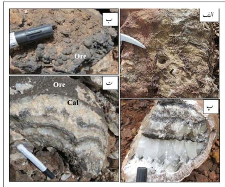
شکل ۵- انواع بافت و ساخت کانسنگ در کانسار منگنز حلب. الف) بافت رگه- رگچه‌ای منگنز و گوتیت در واحد مرمر جان‌گوتاران، ب) بافت خوشه‌ای کانی پیرولوژیت، پ) نمایی از کانه‌زایی منگنز همراه با کلسیت‌های گرمابی با بافت شانه‌ای، ت) کانه‌زایی به صورت بافت گل‌کلمی (کلوفرمی) همراه با کربنات‌های گرمابی. (Cal: کلسیت، Ore: ماده معدنی).
