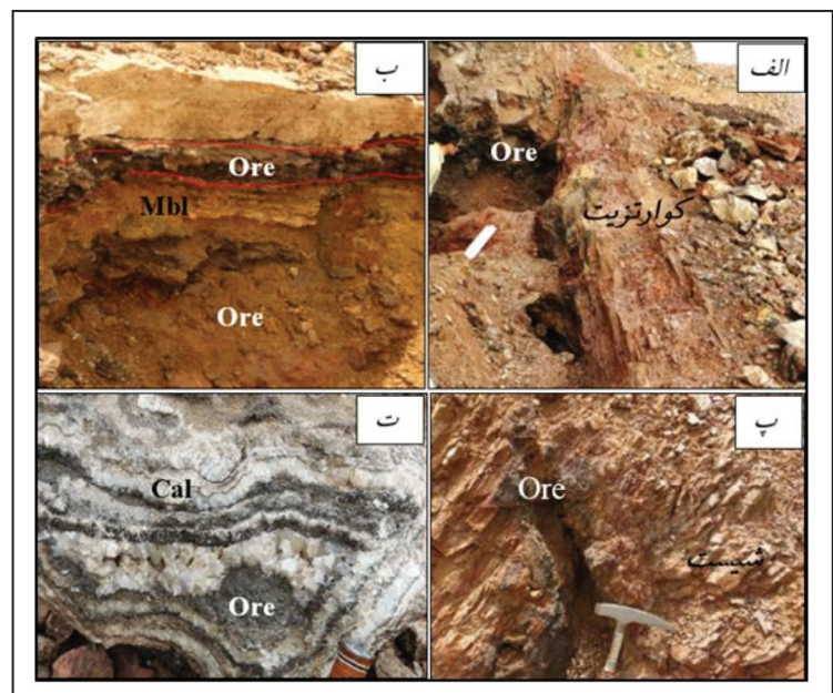
شکل ۴- الف) نمایی از کانه‌زایی منگنز حلب به‌صورت رگه‌ای در داخل واحدهای شیستی و کوارتزی، ب) نمایی از کانه‌زایی منگنز حلب به‌صورت رگه‌ای در داخل واحد مرمر جان‌گوتاران، پ) نمایی از رگه منگنز در واحد مسکویت شیست، ت) نمایی نزدیک از کانه‌زایی منگنز به‌همراه کلسیت گرمابی که دارای بافت دندان‌سگی هستند. (Cal: کلسیت، Mbl: مرمر، Ore: ماده معدنی).
