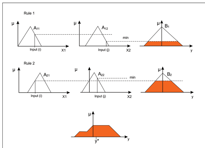
شکل ۴- مدل‌های گرافیکی استنتاج ماکزیمم - مینیمم با ورودی‌های کریسیبی.
