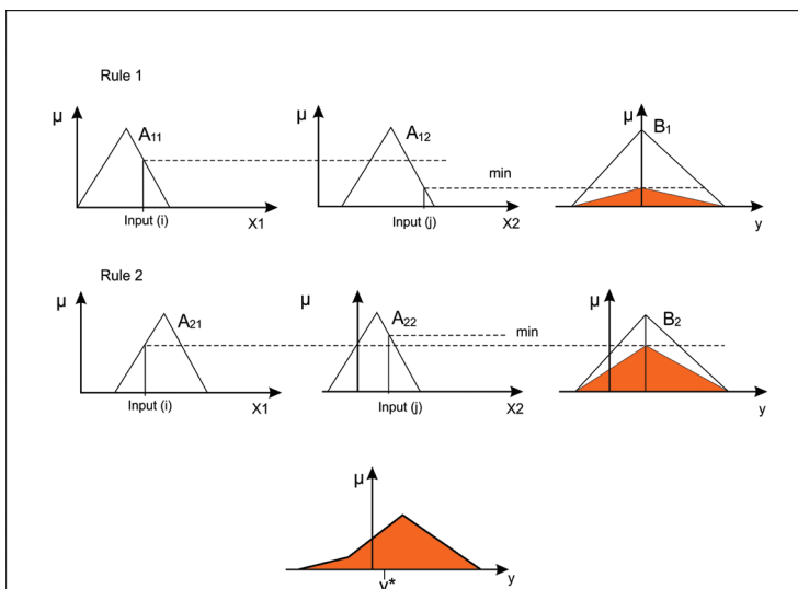
شکل ۵- مدل‌های گرافیکی استنتاج ماکزیمم - ضرب با ورودی‌های کریسیبی.
