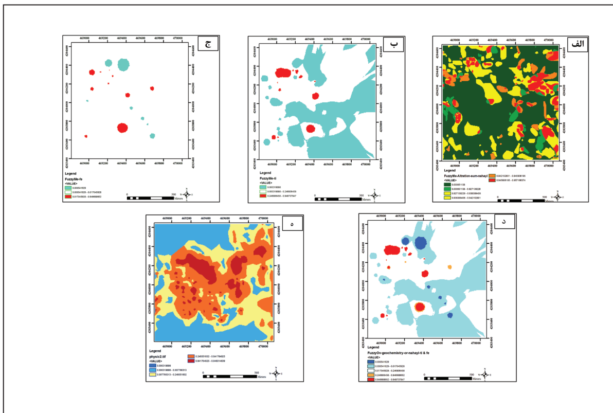
شکل ۷- نقشه‌های فاکتوری منطقه مورد مطالعه: الف) فاکتور دگرسانی؛ ب) فاکتور عیار تیتانیوم؛ ج) فاکتور عیار آهن؛ د) فاکتور ژئوشیمی حاصل از روش تلفیق با استفاده از عملگر OR؛ ه) فاکتور ژئوفیزیکی.
