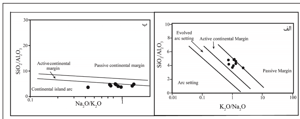
شکل ۸- جایگاه تکتونیکی ماسه‌سنگ‌های سازند قرمز بالایی در بُرش کانسار چهارآباد در نمودارهای (Roser and Korsch 1986)
