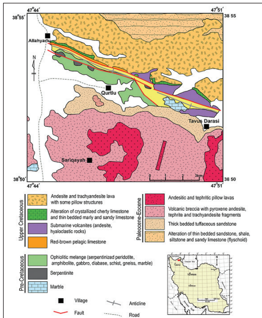
شکل ۱- نقشه زمین‌شناسی ۱:۱۰۰۰۰۰ منطقه الهیارلو اقتباس از نقشه لاهرود (باباخانی و خان‌ناظر، ۱۳۷۰).
