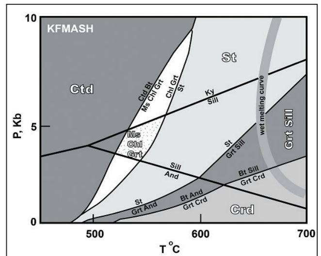
شکل ۶- تخمین فشار با استفاده از شبکه پتروژنتیکی (Holland and Powell, 1998).
