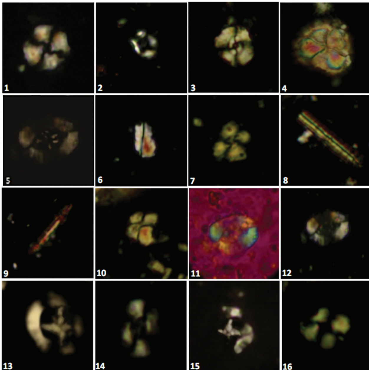
پلیت ۲- تصاویر میکروسکوپ نوری برخی از نانوفسیل‌های آهکی شناسایی شده با بزرگنمایی 1250X.
