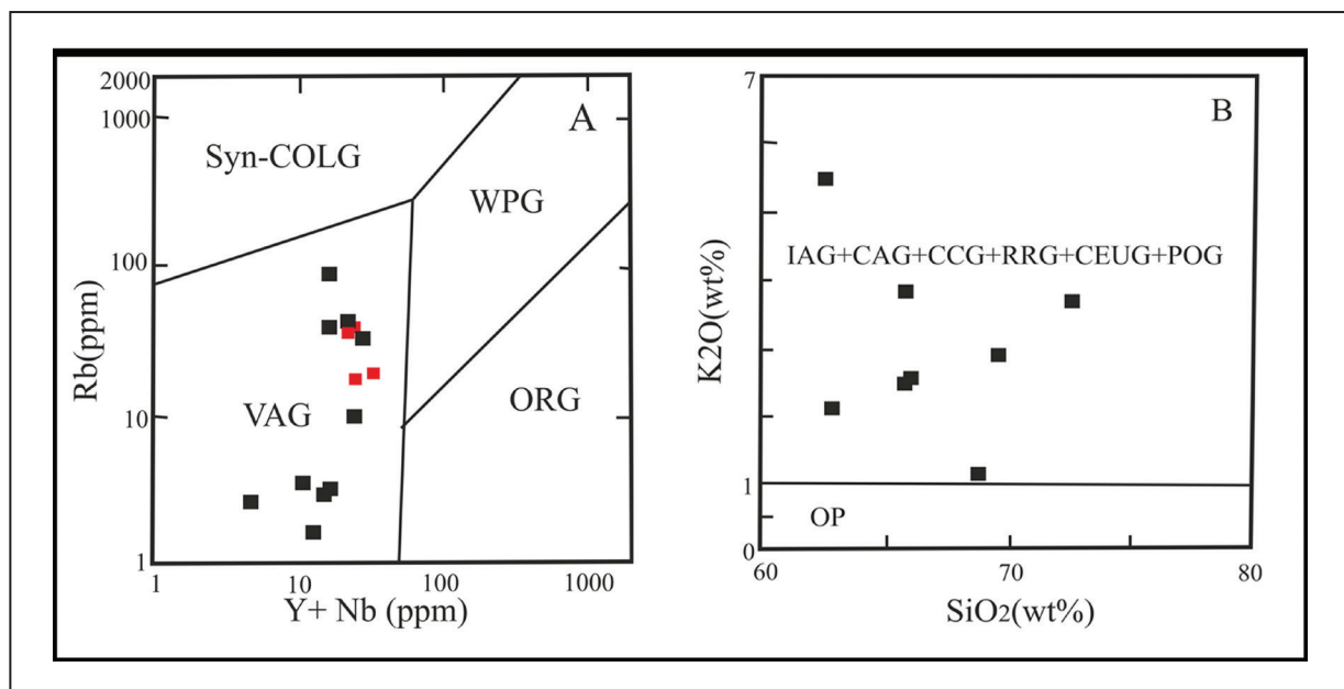
شکل ۸- خاستگاه گرانیتوئیدهای صاحب در نمودارهای تکنونیک (Pearce et al., 1984). نمونه‌های قرمز رنگ از عابادی (۱۳۸۶).
