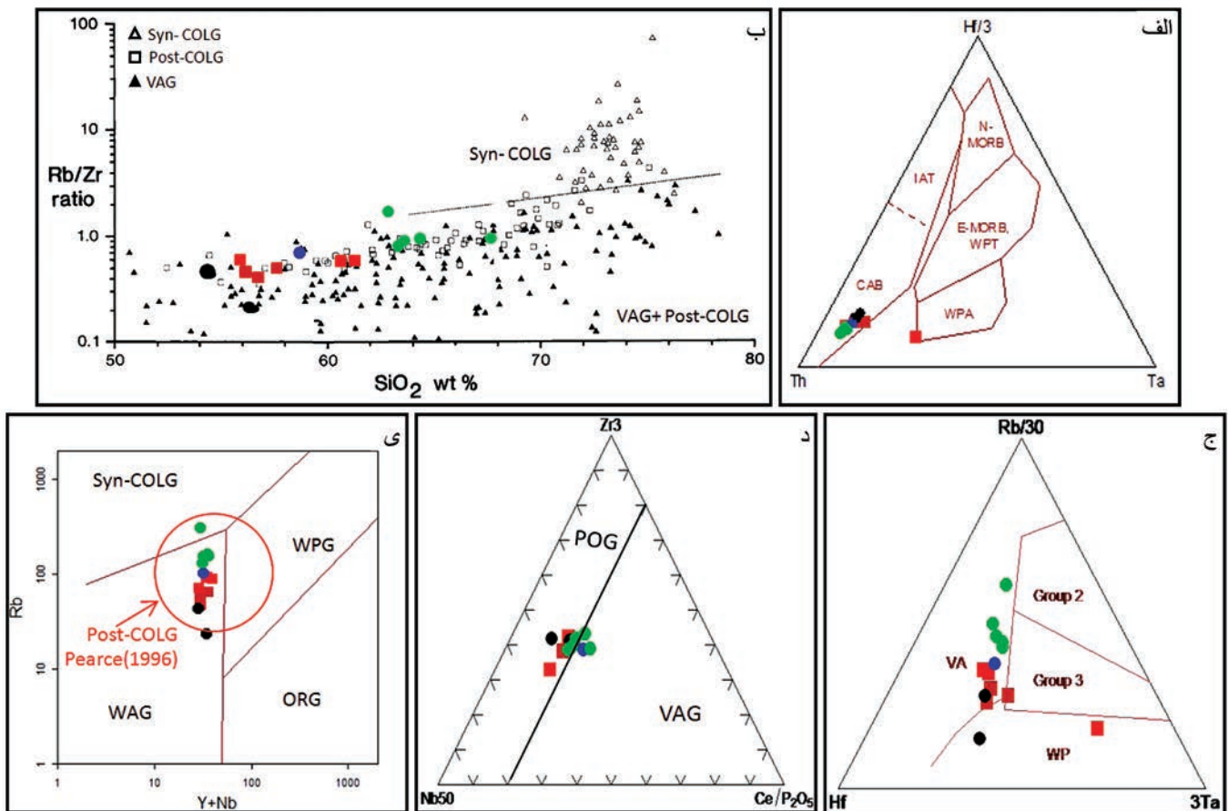
شکل ۱۳- نمودارهای تعیین موقعیت زمین‌ساختی نمونه‌های آتشفشانی، آتشفشانی - نیمه آتشفشانی و نیمه نفوذی محدوده ماهر: الف) نمودار Th-Hf-Ta پیشنهادی (Wood 1980) که آندزیت‌ها و دیگر سنگ‌های آذرین ماهر در محدوده کمان آتشفشانی قرار می‌گیرند؛ ب و ج) نمودارهای پیشنهادی (Harris et al., 1986): نمودار SiO_2 در برابر Rb/Zr و نمودار Rb/30-Hf-Ta*3 که در این نمودارها، نمونه‌ها بیشتر با تمایلی مشخص به سوی جایگاه پس‌برخوردی قرار گرفته‌اند؛ د) نمودار Zr*3-Nb*50-Ce/P2O5 پیشنهادی (Muller & Groves 1997) که در آن نمونه‌ها در محدوده کمان‌های پس از برخورد قرار می‌گیرند؛ ی) نمودار Y+Nb در برابر Rb (Pearce et al., 1984) با محدوده پیشنهادی (Pearce 1996) برای توده‌های پس‌برخوردی که بر پایه آن، این سنگ‌ها در محدوده پس از برخورد تشکیل شده‌اند.
