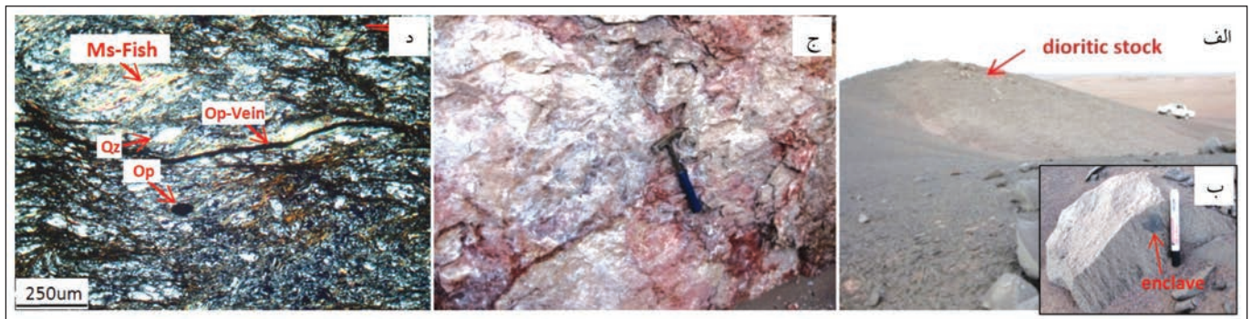
شکل ۲- الف) نمای از استوک میکرودیوریتی؛ ب) آنکلاو مافیک موجود در کوارتز دیوریت همان استوک؛ ج) آینه گسل امتدادلغز راست‌بر؛ د) نمای از میکا ماهی و کوارتزهای طولیل شده، با سوی راست‌بر (XPL). Ms-Fish: میکا (موسکوویت) ماهی، Qtz: کوارتز، Op: کانی اپک.
