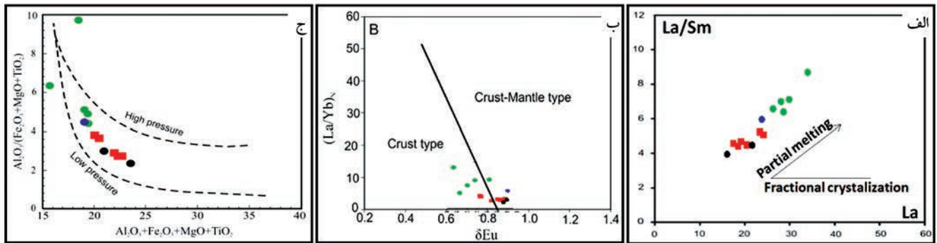
شکل ۱۲- الف) نمودار La در برابر La/Sm (Li et al., 2011) که روند ذوب بخشی و نه تفریق را برای تکامل ماگمای مادر سنگ‌های آذرین ماهر نشان می‌دهد؛ ب و ج) نمودار \delta Eu در برابر (La/Yb)_n (Zhang et al., 2014) و نمودار (Geng et al., 2009) که بیانگر نقش مشترک گوشته و پوسته در تشکیل ماگمای مادر سنگ‌های محدوده ماهر است.
