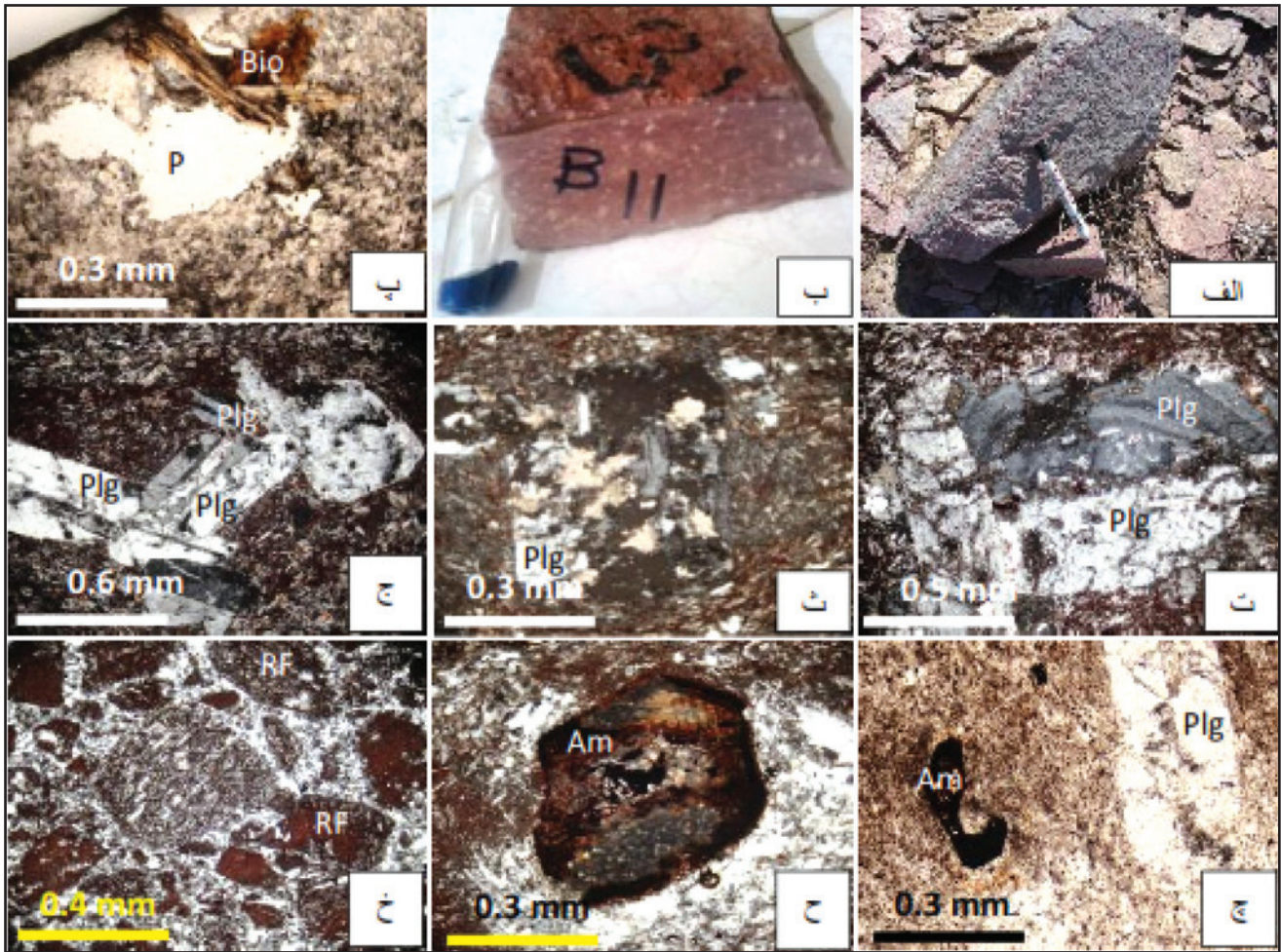
شکل ۳- تصاویر نمونه دستی و میکروسکوپی از سنگ‌های آتشفشانی شمال خاور تالاب گاوخونی. الف) ساخت جریان‌های ریولیتی؛ ب) تصویر نمونه دستی از تراکی داسیت دارای درشت‌بلورهای پلاژیوکلاز سفیدرنگ در زمینه دانه‌ریز تا شیشه‌ای؛ پ) بافت گلومروپرفیریتیک (تجمع بلورهای بیوتیت) و بافت ویزیکولار در تراکی داسیت؛ ت) بافت گلومروپرفیریتیک (تجمع بلورهای پلاژیوکلاز) در تراکی آندزیت؛ ث) جانشینی بلورهای پلاژیوکلاز از حاشیه‌ها توسط کانی‌های کربناتی در تراکی آندزیت؛ ج) بلورهای درشت پلاژیوکلاز غربالی شده در تراکی آندزیت؛ چ) خوردگی خلیجی در بلور آمفیبول اابسیت شده و نفوذ خمیره سنگ در بلور پلاژیوکلاز در تراکی آندزیت؛ ح) مقطع عرضی بلور آمفیبول خورده و اابسیت شده در تراکی آندزیت؛ خ) قطعات خرده‌سنگی اسیدی تا حدواسط فراوان در توف خرده سنگی. تصاویر پ و چ در نور PPL و دیگر تصاویر میکروسکوپی در نور XPL گرفته شده‌اند. Bio: بیوتیت، P: حفره، plg: پلاژیوکلاز، Am: آمفیبول، RF: خرده سنگ آتشفشانی. نشانه‌های اختصاری کانی‌ها از Kretz (1983) گرفته شده‌اند.
