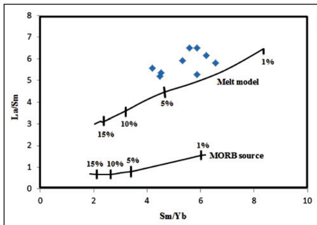
شکل ۲۴- نمودار La/Sm - Sm/Yb ، برای تعیین مدل ذوب بخشی تعادلی در گوشته غنی شده و مورب تهی شده. نمودار پایه از Sun & McDonough (1989) است. نمونه‌های منطقه مورد مطالعه، بیشتر درجات ذوب بخشی تعادلی ۱ تا ۵ درصدی از یک منشأ غنی شده را نشان می‌دهند.
