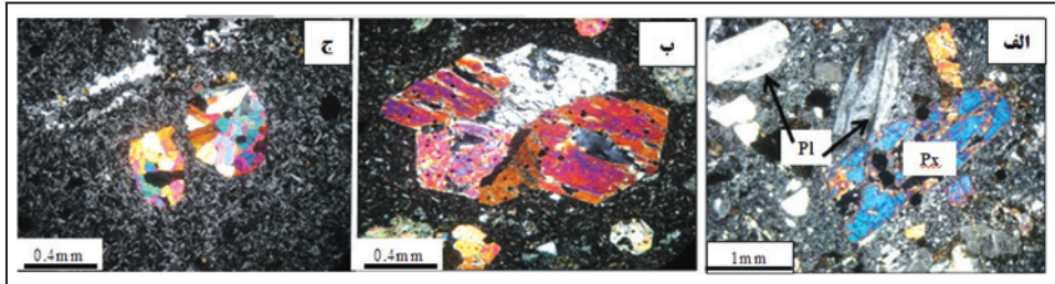
شکل ۱۲- الف) تصویر میکروسکوپی از بازالت‌های دشت کوه که بافت پورفیری را در این سنگ نشان می‌دهد. شکستگی و ادخال از کانی‌های ثانویه و کدر را در کانی پیروکسن به خوبی می‌توان دید؛ ب) تصویر میکروسکوپی از بافت گلوپورفیری و تجمع کانی‌های پیروکسن در بازالت‌های دشت کوه؛ ج) تصویر میکروسکوپی از بافت بادامکی در بازالت‌های دشت کوه. حفره‌ها توسط کانی‌های ثانویه کلریت و اپیدوت پر شده است. زمینه این سنگ، شامل ریزبلورهای پلاژیوکلاز است. همه تصاویر در نور پلاریزه متقاطع با بزرگنمایی ۴۰ برابر تهیه شده‌اند.
