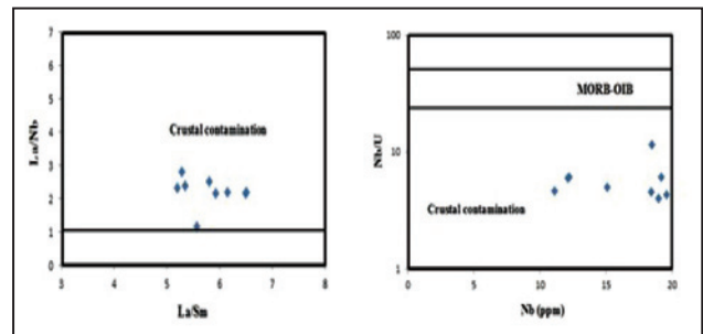
شکل ۲۳- موقعیت نمونه‌های مورد مطالعه روی نمودارهای La/Nb در برابر La/Sm و Nb/U در برابر Nb برای U . نمودار پایه از Yan & Zhao (2008) است. این نمودارها، نقش آرایش پوسته‌ای را در تشکیل این سنگ‌ها اثبات می‌کنند.
