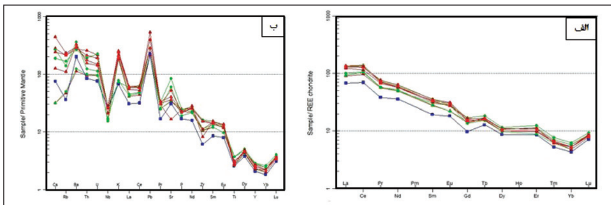
شکل ۱۸- الف) نمودار عناصر خاکی کمیاب سنگ‌های منطقه مورد مطالعه، به‌نحی که با کندریت (Boynton, 1984) مقایسه شده است؛ ب) نمودار عنکبوتی برای مقایسه عناصر فرعی و کمیاب سنگ‌های منطقه مورد مطالعه، به‌نحی که با گوشته اولیه (Sun & McDonough, 1989) مقایسه شده است (نمادها همانند شکل ۱۵).
