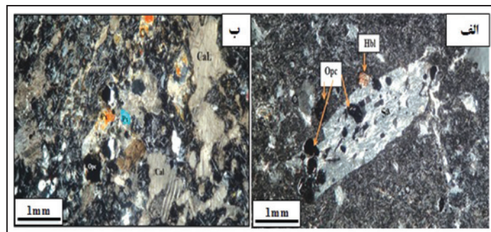
شکل ۱۲- الف) تصویر میکروسکوپی از بازالت‌های دشت کوه که بافت پورفیری را در این سنگ نشان می‌دهد. شکستگی و ادخال از کانی‌های ثانویه و کدر را در کانی پیروکسن به خوبی می‌توان دید؛ ب) تصویر میکروسکوپی از بافت گلوپورفیری و تجمع کانی‌های پیروکسن در بازالت‌های دشت کوه؛ ج) تصویر میکروسکوپی از بافت بادامکی در بازالت‌های دشت کوه. حفره‌ها توسط کانی‌های ثانویه کلریت و اپیدوت پر شده است. زمینه این سنگ، شامل ریزبلورهای پلاژیوکلاز است. همه تصاویر در نور پلاریزه متقاطع با بزرگنمایی ۴۰ برابر تهیه شده‌اند.
