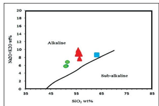
شکل ۱۹- موقعیت سنگ‌های آتشفشانی دشت‌کوه در نمودار TAS، به منظور تعیین سری ماگمایی؛ همه نمونه‌ها در سری ماگمایی آکالن قرار می‌گیرند. نمودار پایه از Irvine & Baragar (1971) است (نمادها همانند شکل ۱۵).
