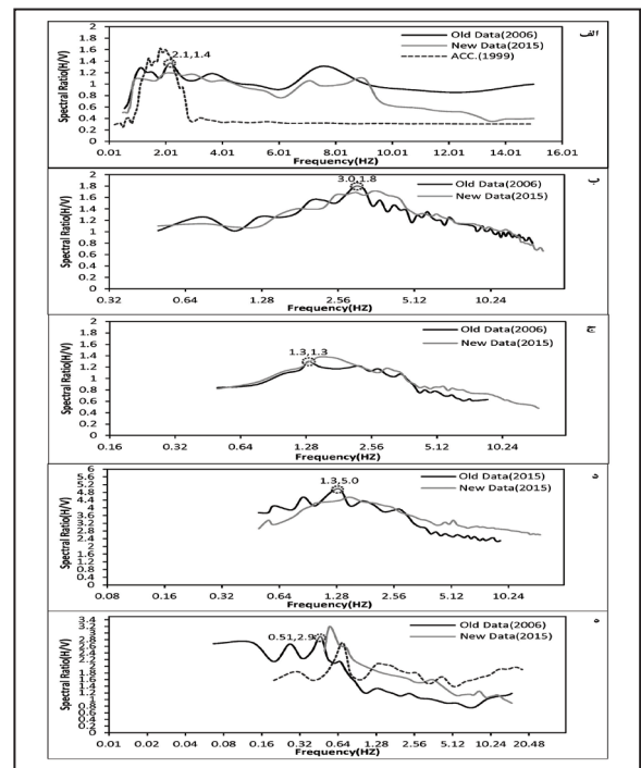
شکل ۱- الف) نمودار نسبت طیفی در ایستگاه ۱۲S؛ ب) نمودار نسبت طیفی در ایستگاه ۲۳S؛ ج) نمودار نسبت طیفی در ایستگاه ۳۳S؛ د) نمودار نسبت طیفی در ایستگاه ۴۳S؛ ه) نمودار نسبت طیفی در ایستگاه ۴۴S.
