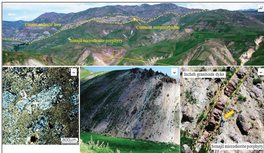
شکل ۲- الف) نفوذ توده میکرودیوریت پورفیری سوناجیل به درون واحدهای گدازه ای انوسن، با حاشیه دگرگون شده؛ ب) نفوذ دایک هایی از توده گرانیتویدی اینچه به درون توده پورفیری سوناجیل، پ) تصویر بزرگ شده از توده پورفیری سوناجیل که به شدت دگرسان شده است؛ ت) تصویر میکروسکوپی از توده پورفیری سوناجیل، که تحت تأثیر سرسیتی شدن قرار گرفته است (Plg: پلاژیوکلاز).
