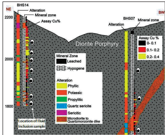
شکل ۶- الف) نمودار گل‌سرخ‌ی رگه‌های اصلی کانهدار در کانسار پورفیبری سوناجیل؛ روند کلی رگه‌ها به صورت شمال شمال باختر- جنوب جنوب خاور است؛ ب) نیم‌رخ زمین‌شناسی روی توده میکرودیوریت پورفیبری میزبان کانی‌زایی در جهت شمال خاور- جنوب باختر بر پایه گمانه‌های BSH07 و BSH14، که روی آن پهنه‌های کانی‌زایی، دگرسانی و تغییرات عیار مس به همراه محل نمونه‌برداری میانبرهای سیال مشخص شده است (حسین زاده، ۱۳۸۷).
