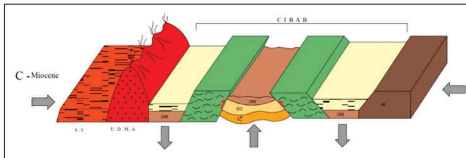
شکل ۹- فرایش حوضه رسوبی تلمسی تحت تأثیر عملکرد گسل‌های کنترل‌کننده آن و سامانه فشارشی حاکم بر کل ایران مرکزی (شایانفر، ۱۳۹۳).
