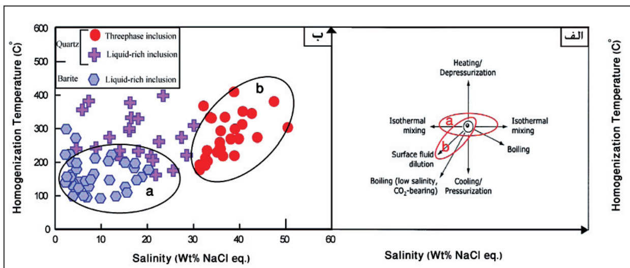
شکل ۸- الف) نمودار نمادین جهات اصلی دمای همگن‌شدگی - شوری در طی فرایندهای مختلف تکامل میانبارهای سیال (Wilkinson, 2001); ب) نمودار دمای همگن‌شدگی - شوری میانبارهای سیال کانسار همیرد.
