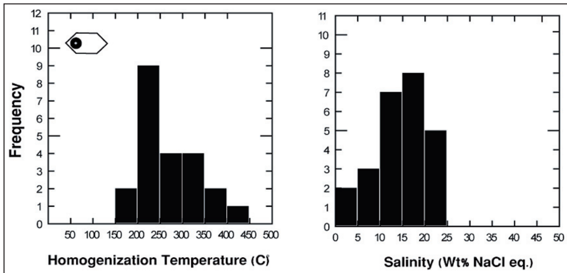
شکل ۶- نمودار ستونی (هیستوگرام) دمای همگن‌شدگی و شوری میانبارهای سیال دوفازی غنی از مایع درکانی کوارتز.
