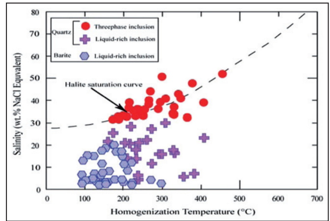
شکل ۹- نمودار دمای همگن‌شدگی- شوری میانبارهای سیال کانسار آهن همیرد.
