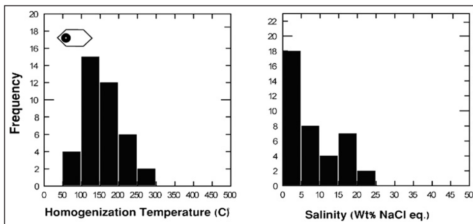
شکل ۷- نمودار ستونی دمای همگن‌شدگی و شوری میانبارهای سیال دوفازی غنی از مایع درکانی باریت.
