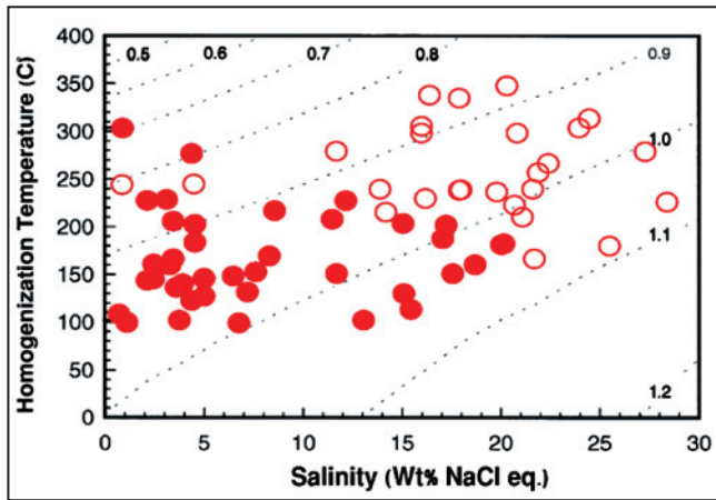
شکل ۱۰- نمودار شوری-دمای همگن‌شدگی میانبارهای سیال نمونه‌های کانسار همیرد برای تعیین چگالی (Wilkinson, 2001)؛ دایره تو پر: میانبار سیال دوفازی کانی باریت؛ دایره تو خالی: میانبار سیال دوفازی کانی کوآرتز.
