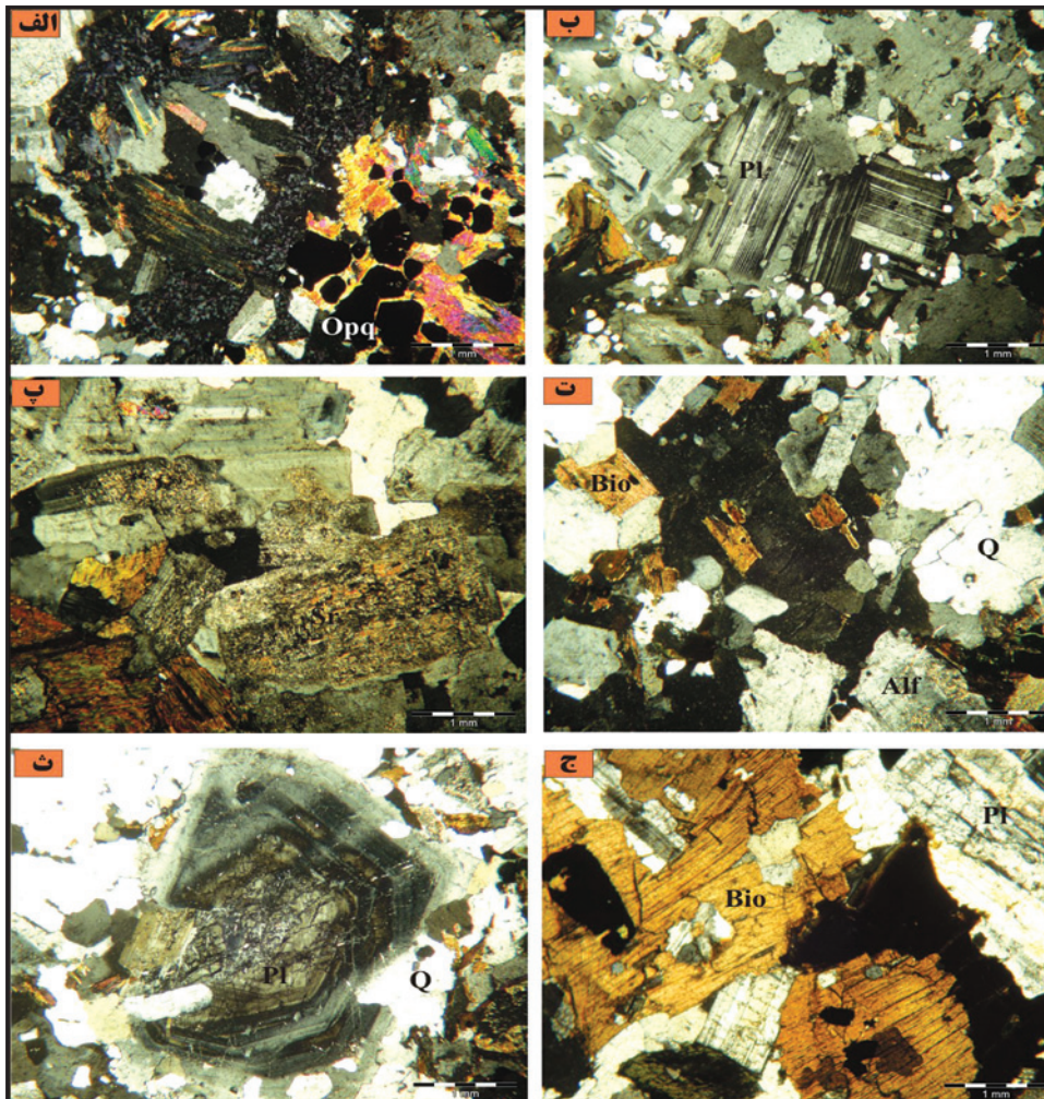
شکل ۳- الف) فراوانی کانی‌های مافییک و کیدر در کوارتزدیوریت؛ ب) ماکل پلی‌سنتیک در گرانودیوریت؛ پ) دگرسانی بلورهای پلاژیوکلاز به سریسیت و اپیدوت در گرانودیوریت؛ ت) نمایی از گرانیت‌های منطقه مورد مطالعه؛ ث) منطقه بندی در گرانیت؛ ج) بیوتیت‌های فراوان گرانیت (Opq): کانی‌های کیدر؛ Pl: پلاژیوکلاز؛ Sr: سریسیت؛ Q: کوارتز؛ Bio: بیوتیت؛ Alf: فلدسپار قلیایی) (همه شکل‌ها در نور پلاریزه متقاطع (Xpl) برداشت شده‌اند.
