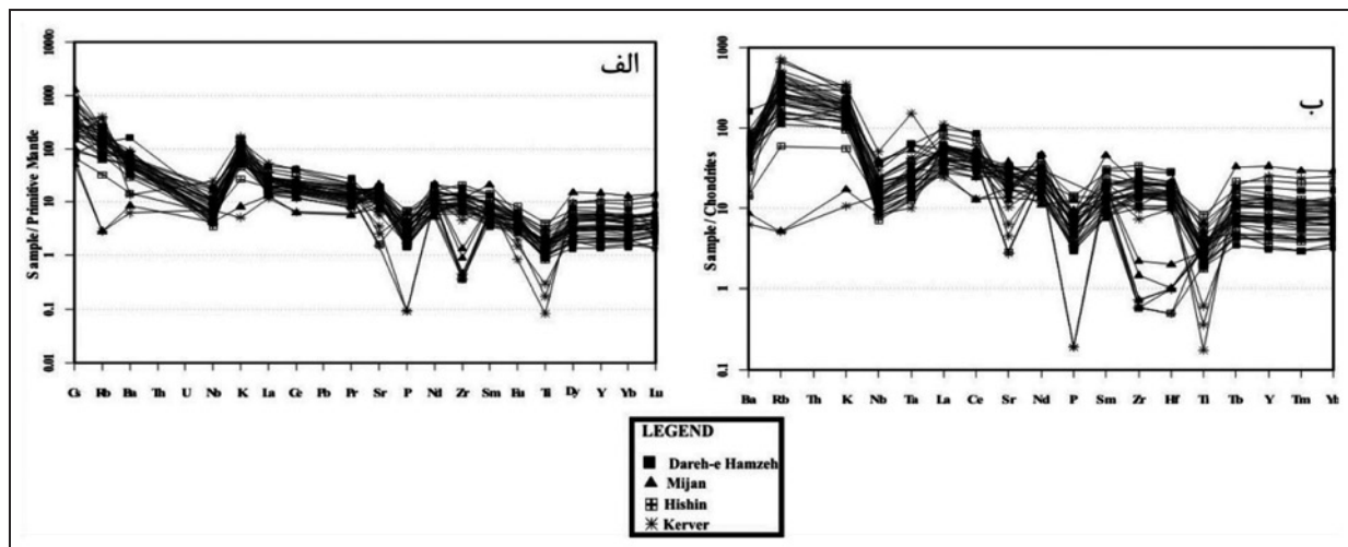
شکل ۸- الف) نمودار بهنجار شده بر پایه گوشته اولیه؛ ب) نمودار بهنجار شده بر پایه کندریت.
