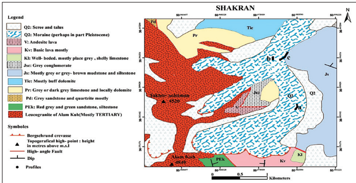
شکل ۳- نقشه زمین‌شناسی منطقه برداشت و موقعیت پروفیل‌های برداشتی GPR برگرفته از (Annells et al. 1977).
