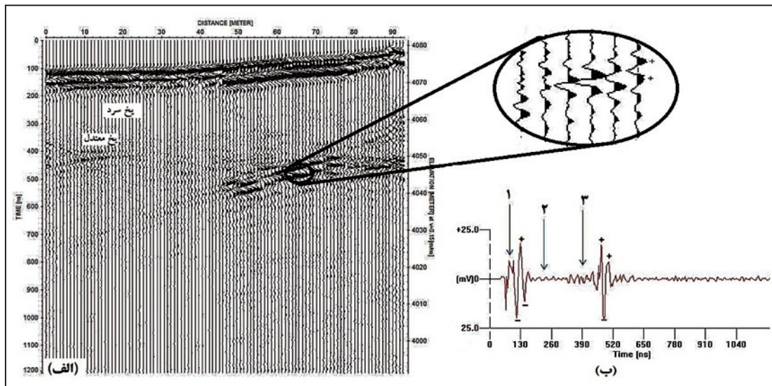
شکل ۵- الف) مقطع ژرفی پروفیل a پس از پردازش‌های تصحیح اشباع سیگنال، تصحیح استاتیک، تابع تقویت و تصحیح توپوگرافی؛ ب) رد واقع در فاصله ۶۲ متری ابتدای پروفیل با حادثه‌ها و ناحیه‌های مشخص شده روی آن.
