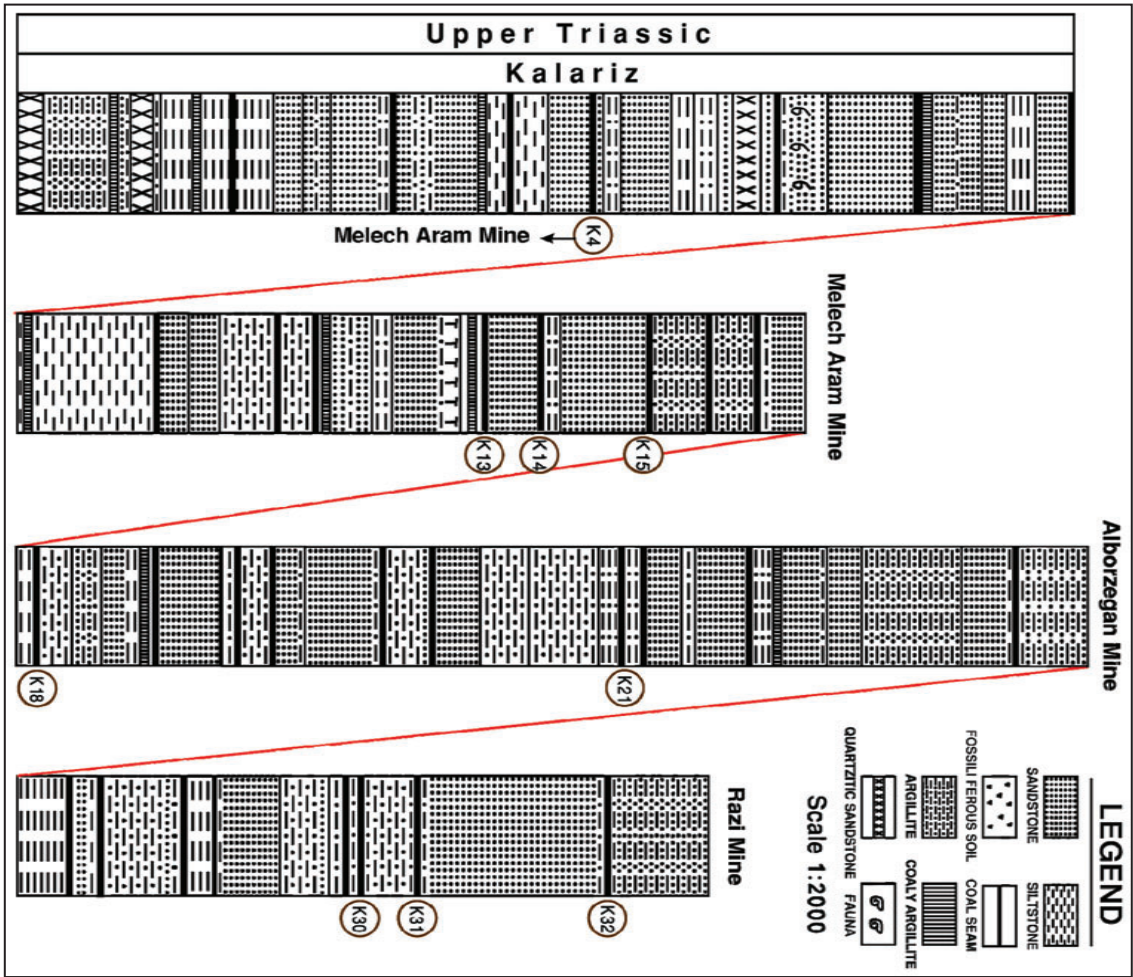
شکل ۳- ستون چینه‌شناسی لایه‌های زغال سنگی منطقه اولنگ که لایه‌های مورد مطالعه بر روی آن مشخص شده‌اند (زیسی، ۱۳۷۲).
