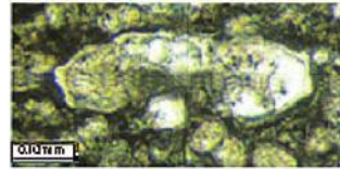
Globotruncana bulloides
