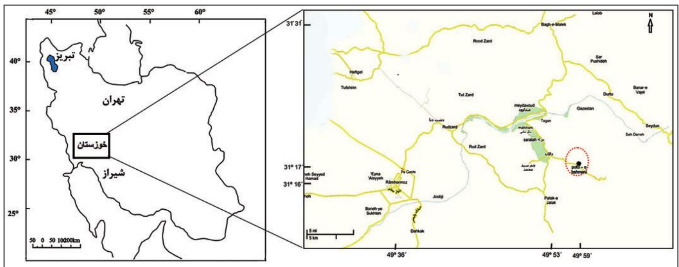
شکل ۱- موقعیت جغرافیایی و راه دسترسی به برش مورد مطالعه
