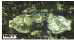
Marginotruncana coronata
