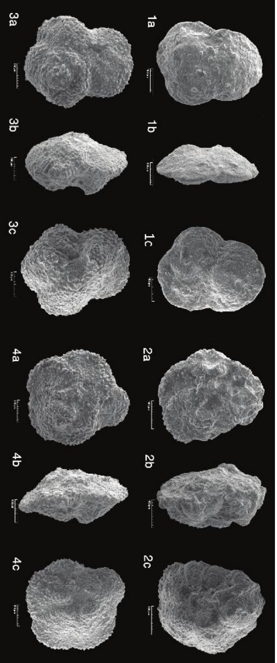
1- Globanomalina pseudomenardii ×100µm 2- Morozovella velascensis ×100µm 3- Morozovella aequa ×100µm 4- Morozovella oclusa ×100µm
