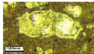
Globotruncana lapparenti
