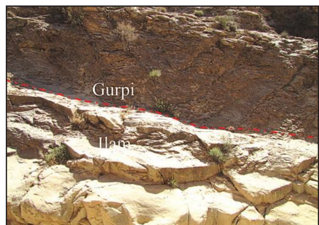
شکل ۲- نمایی از مرز پایینی سازند گورپی با سازند ایلام در برش کوه سفید
