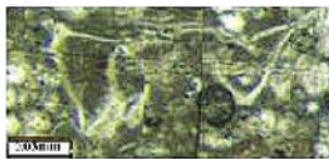
Dicarinella asymetrica
