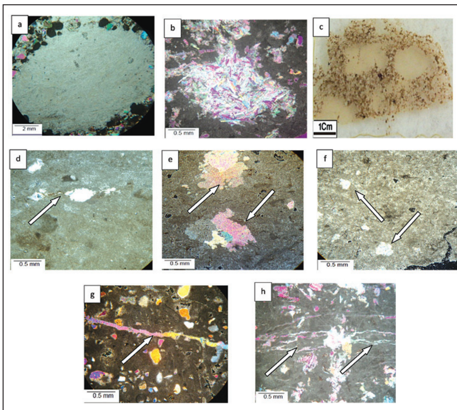
شکل ۴- (a) انیدریت گرهکی در ماسه سنگ، چاه شماره ۴۸ با ژرفای ۲۱۹۴ متری؛ (b) انیدریت گرهکی در دولستون، چاه شماره ۴۸ با ژرفای ۲۱۸۹/۴ متری (نور XPL)؛ (c) انیدریت گرهکی با بافت قفس مرغی، چاه شماره ۴۸ با ژرفای ۲۱۹۴/۹۰ متری؛ (d) انیدریت گرهکی تدفینی در امتداد استیلولیت، چاه شماره ۴۸ با ژرفای ۲۱۸۸/۲۰ متری (نور XPL)؛ (e) و (f) انیدریت پراکنده و منفرد، چاه شماره ۴۸، (e) با ژرفای ۲۱۸۶/۴۷ متری و (f) با ژرفای ۲۱۸۵ متری (نور XPL)؛ (g) انیدریت پراکنده شکستگی، چاه شماره ۴۷ با ژرفای ۲۱۸۹ متری (نور XPL)؛ (h) انیدریت رگچه‌ای، چاه شماره ۴۸ با ژرفای ۲۱/۴ متری (نور XPL).
