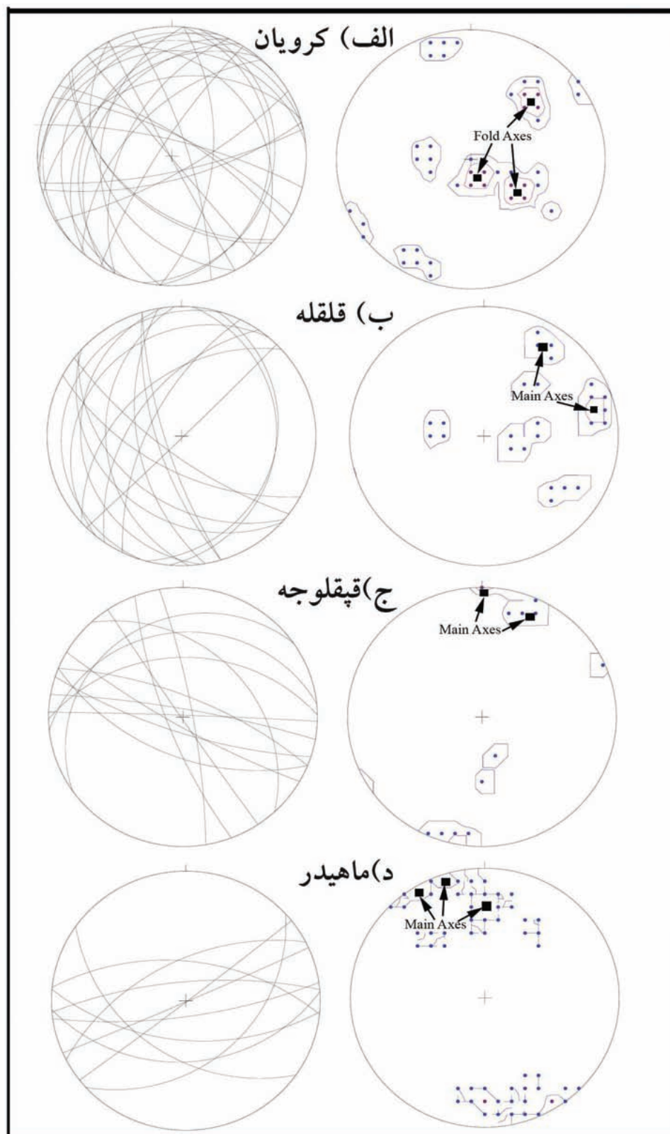
شکل ۸- محاسبه سطوح محوری و محور ریزجین‌های تشکیل شده در فاز شکل‌پذیر و نیمه‌شکل‌پذیر در بخش‌های باختری (ایستگاه‌های کرویان، قلقله و قیقلوجه) و مرکزی (ایستگاه ماهیدر).
