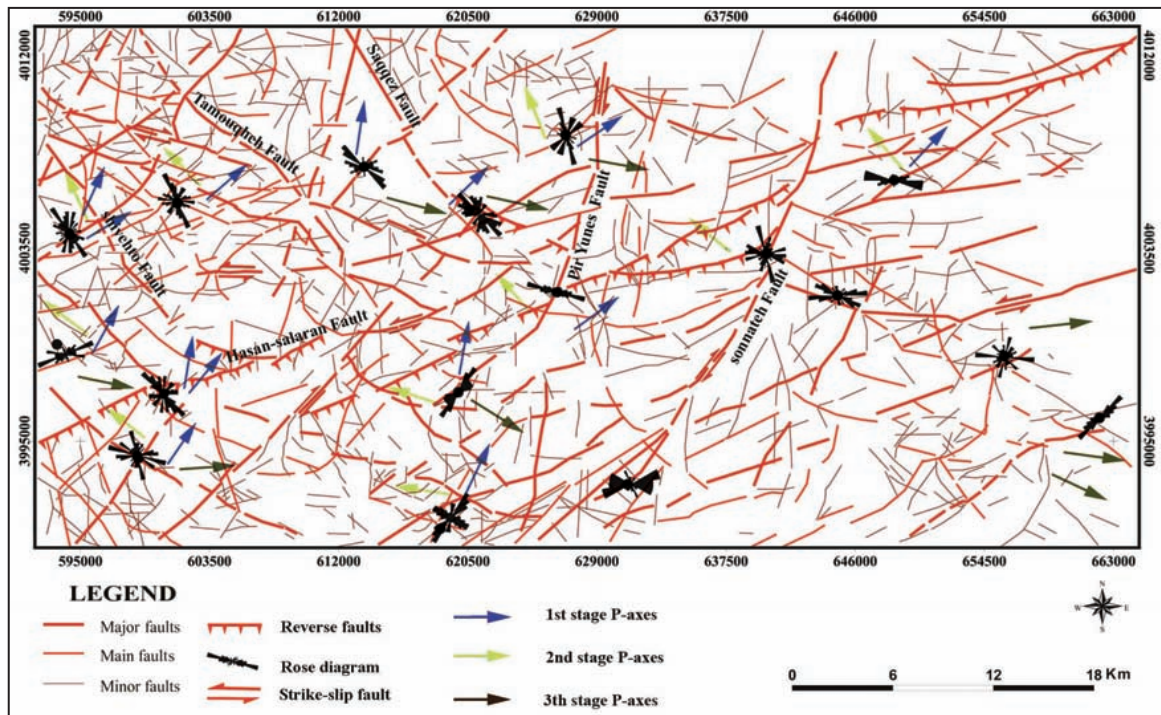
شکل ۴- نقشه ساختاری منطقه مورد مطالعه شامل ساختارهای استخراج و پیمایش شده، به همراه نمودارهای گل سرخی و محورهای فشارش در ایستگاه‌های مختلف اندازه‌گیری (نسل‌های مختلف محورها با رنگ‌های متفاوت نمایش داده شده‌اند).
