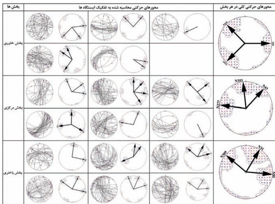
شکل ۱۳- محورهای فشارشی به دست آمده در سه بخش خاوری، مرکزی و باختری و کلی هر بخش.
