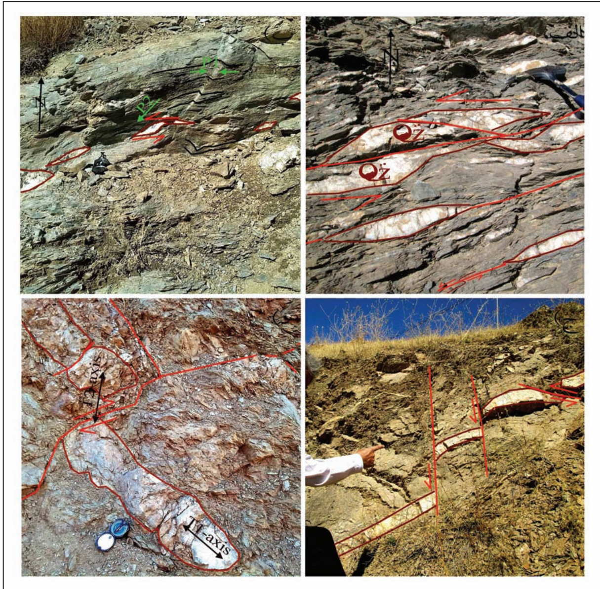
شکل ۶- نماهایی از گسلش در محیط‌های شکل‌پذیر تا شکننا: الف) ایجاد پهنه برشی چپ‌بر در محیط شکل‌پذیر که در ادامه نیز دوباره با این سازوکار به صورت نیمه‌شکل‌پذیر بریده شده است؛ ب) نمایی از چین‌خوردگی در شکل‌پذیر (نسل اول حرکت P1) که در ادامه توسط یک پهنه برشی در محیط شکل‌پذیر (نسل دوم حرکت P2) قطع شده است؛ ج) نمایی از یک بودیناژ که در یک محیط شکننده بریده و جابه‌جا شده است؛ د) نمایی از گسلش در محیطی کاملاً شکننده.
