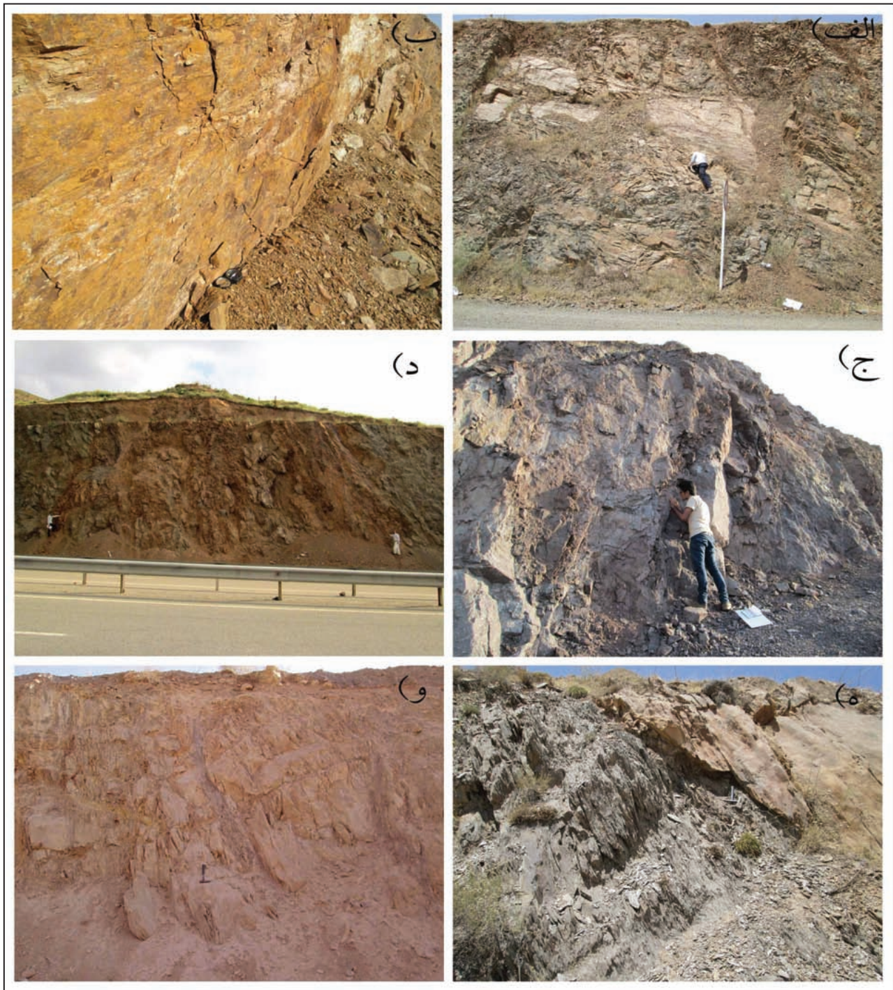
شکل ۷- نمایی از سطوح گسل های اصلی اندازه گیری شده در منطقه مورد مطالعه؛ الف) گسل تموغه در خاور روستای تموغه؛ ب) گسل شیواتو در جنوب باختری روستای شیواتو؛ ج) گسل سقز در جنوب - خاوری شهرستان سقز؛ د) گسل حسن سالاران در شمال خاوری روستای سننه؛ ه) گسل پیرونس در پیرامون روستای درگاه سلیمان؛ و) گسل سننه در خاور روستای سننه.
