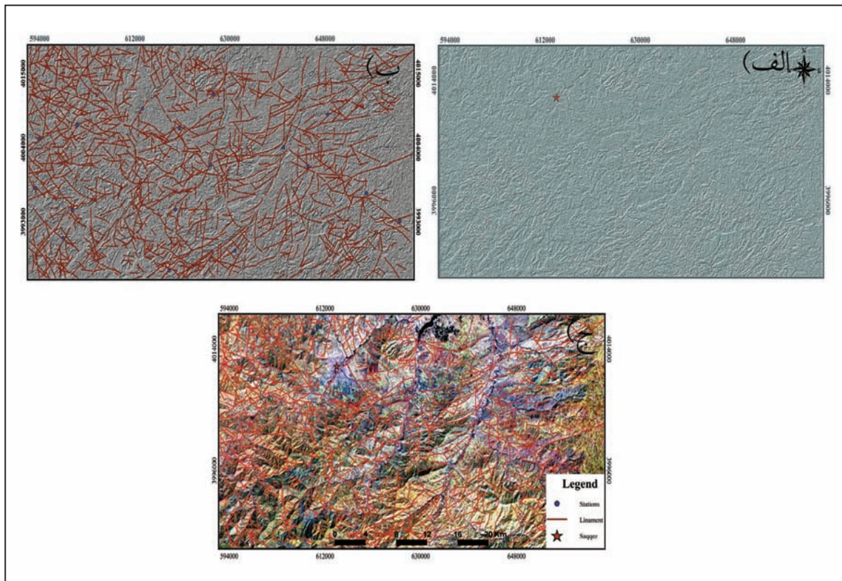
شکل ۳- اعمال فیلتر بر تصویر ماهواره ای ETM+ اصلاح شده و استخراج خطوطها؛ الف) اعمال فیلتر ۴۵ درجه روی باند R تصویر ماهواره ای؛ ب) استخراج عناصر خطی؛ ج) کنترل عناصر خطی از روی تصویر (به همراه پیمایش های صحرائی).
