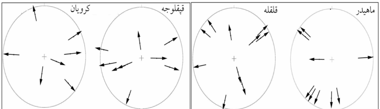
شکل ۱۲- محاسبه محورهای کشش با تحلیل رگه‌های سیلیسی موازی یا متقاطع اندازه‌گیری شده در بخش‌های باختری (ایستگاه‌های کرویان، قیقلوچه و قلقله) و مرکزی (ایستگاه ماهیدر).
