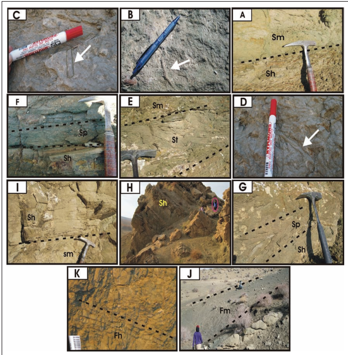
شکل ۲- تصاویر صحرایی انواع رخشاره‌های سنگی در برش‌های مورد مطالعه. (A) رخشاره ماسه‌سنگ توده‌ای (Sm) در برش شوریجه؛ (B، C، D) به ترتیب آثار فسیلی، Paleophycus و Ophiomorpha در ماسه‌سنگ‌های گلاکونیتی توده‌ای بخش زیرین برش باغک؛ (E) رخشاره ماسه‌سنگی دارای چینه‌بندی مورب عدسی شکل (St) در برش شوریجه؛ (F) رخشاره ماسه‌سنگی دارای چینه‌بندی مورب مسطح (Sp) و افقی (Sh) در برش باغک؛ (G) رخشاره ماسه‌سنگی دارای چینه‌بندی مورب مسطح (Sp) در برش شوریجه؛ (H) رخشاره ماسه‌سنگی دارای لایه‌بندی افقی (Sh) در برش باغک (دید به سوی شمال)؛ (I) رخشاره ماسه‌سنگی دارای لایه‌بندی افقی (Sh) و توده‌ای (Sm) در برش شوریجه؛ (J) رخشاره گل‌سنگ توده‌ای (Fm) در برش باغک (دید به سوی جنوب)، K: رخشاره گل‌سنگ لایه‌ای (Fh) در برش شوریجه.
