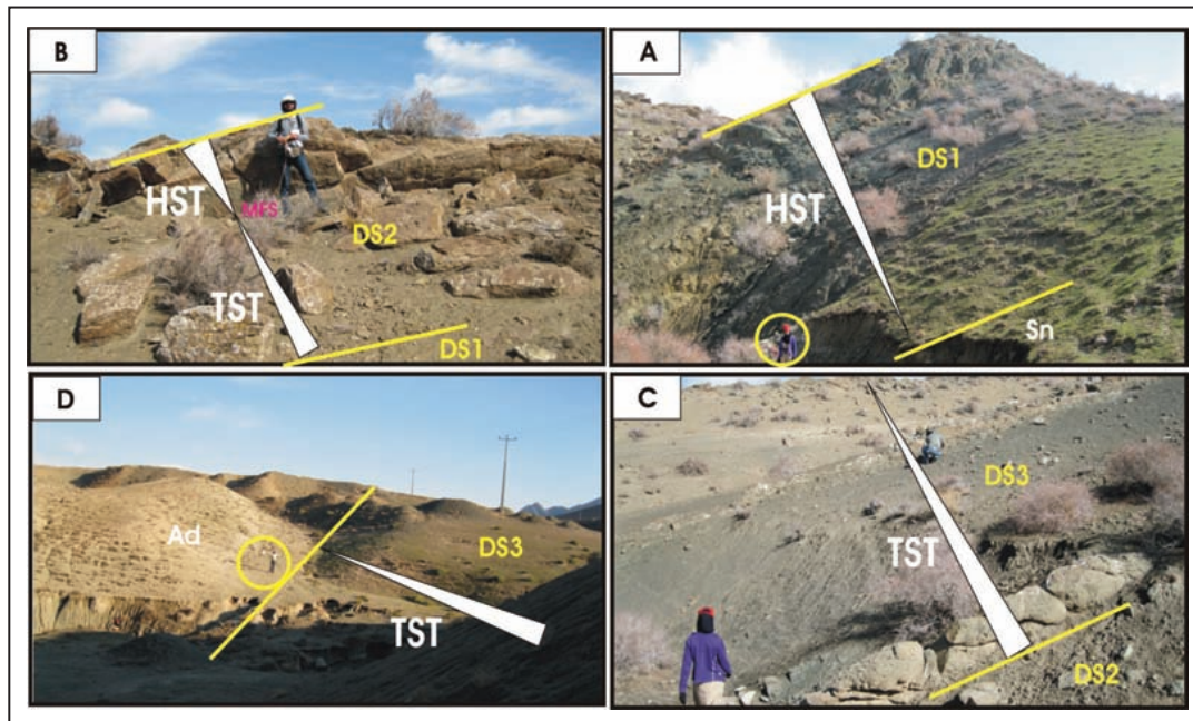
شکل ۶- سکانس‌های رسوبی سازند آیتامیر در برش باغک. (A) دسته‌رخساره HST در سکانس رسوبی اول؛ (B) سکانس رسوبی دوم که شامل دو دسته‌رخساره HST و TST و سطح پیشینه پیشروی (MFS) است؛ (C) سکانس رسوبی سوم که تنها دارای دسته‌رخساره TST است؛ (D) مرز بالایی سکانس رسوبی سوم با سازند آبدراز (Ad) (در همه تصاویر دید به سوی شمال باختر است).
