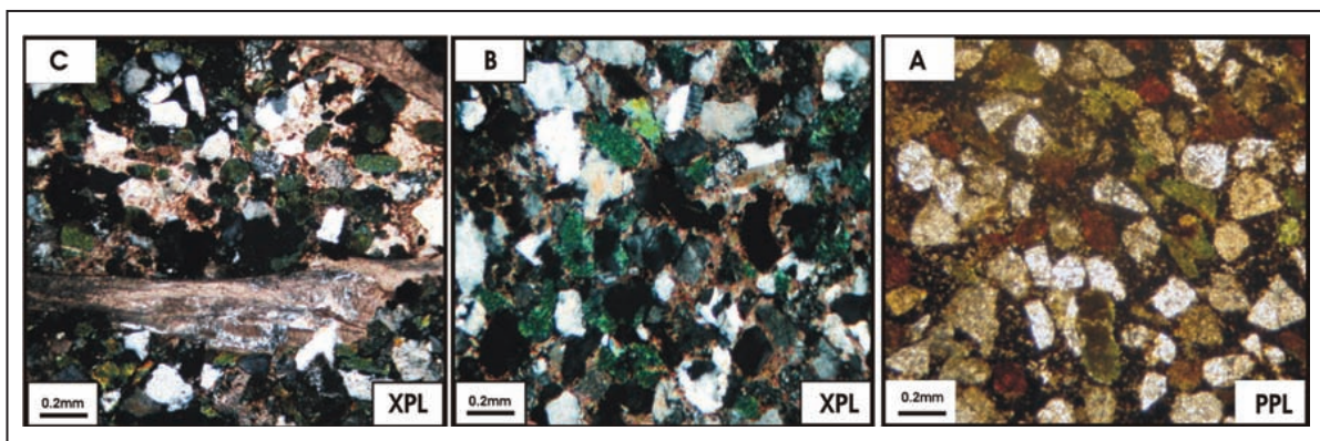
شکل ۳- رخشاره‌های سیلیسی آواری مختلف در برش‌های مورد مطالعه. (A) ساب‌لیتارنایت با جورشدگی خوب ( A_1 )؛ (B) ساب‌آرکوز با جورشدگی متوسط ( A_1 )؛ (C) ساب‌لیتارنایت با جورشدگی ضعیف ( A_2 )
