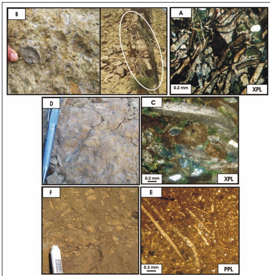
شکل ۴- رخصاره‌های کربناته مختلف در برش‌های مورد مطالعه. (A) رودستون ماسه‌ای بیوکلاستی با گلاکونی و چینه‌بندی مورب (C 1 )؛ (B) رخصاره C 1 در صحرا؛ (C) رودستون ماسه‌ای بیوکلاستی با گلاکونی (C 2 )؛ (D) رخصاره C 2 در صحرا؛ (E) فلوتستون ماسه‌ای بیوکلاستی با آمونیت و گلاکونی (C 3 )؛ (F) رخصاره C 3 در صحرا.
