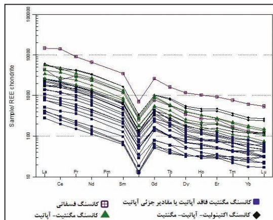
شکل ۱۱- الگوی عناصر خاکی کمیاب نمونه‌های مربوط به کانسنگ مگنتیت-آپاتیت، کانسنگ مگنتیت بدون آپاتیت یا دارای مقادیر جزئی آپاتیت، کانسنگ فسفاتی و کانسنگ اکتینولیت-آپاتیت-مگنتیت (مقادیر بهنجارسازی از (McDonough and Sun (1995)).
