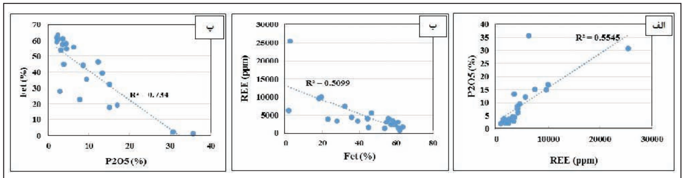
شکل ۱۰- الف) نمودار فراوانی \sum REE در برابر P_2O_5 ؛ ب) نمودار فراوانی Fe در برابر \sum REE؛ پ) نمودار فراوانی Fe در برابر P_2O_5 .
