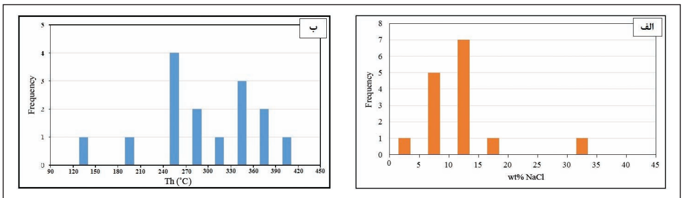
شکل ۱۵- الف) نمودار ستونی فراوانی‌های اندازه‌گیری شده در میانبراهای سیال دوفازی (L+V) که به فاز مایع همگن شده‌اند؛ ب) نمودار ستونی فراوانی محدوده دمایی همگن‌شدگی میانبراهای سیال دوفازی (L+V) که به فاز مایع همگن شده‌اند (L+V→L).
