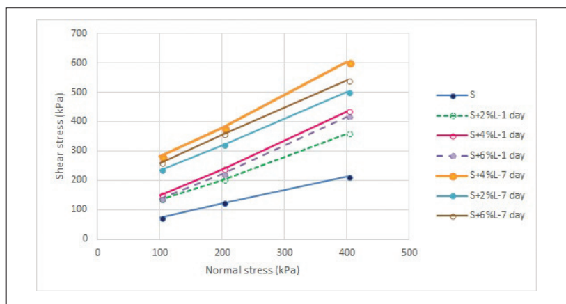
شکل ۳- پوش گسیختگی خاک تثبیت شده با درصد‌های مختلف آهک با ۱ و ۷ روز عمل‌آوری و غیر مسلح.
