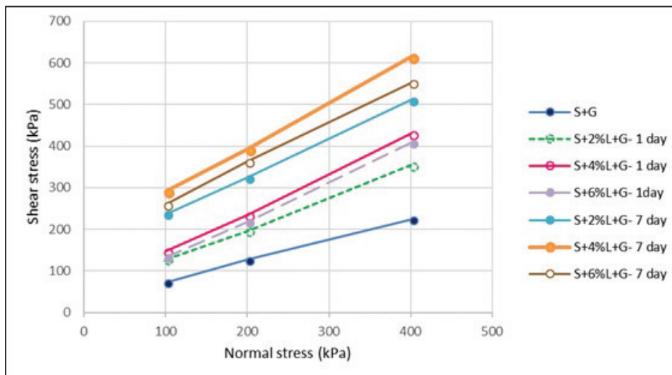
شکل ۷- پوش گسیختگی خاک تثبیت شده با درصدهای مختلف آهک با ۱ و ۷ روز عمل آوری و مسلح شده با ژئوگرید ۱۰×۱۰ میلی متر بدون المان‌های متقاطع عرضی
