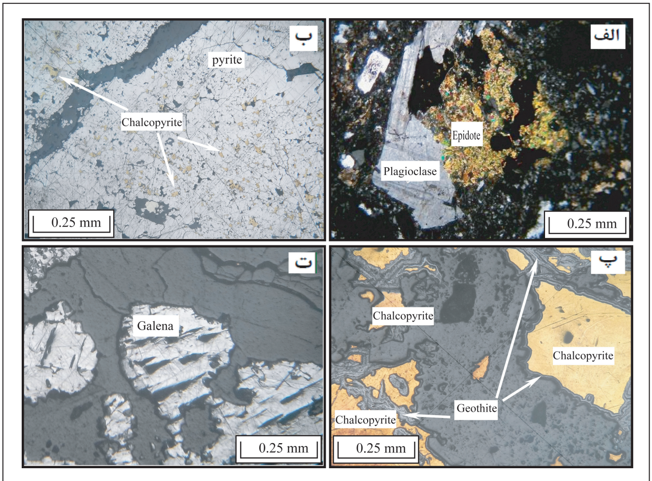
شکل ۴- تصاویر میکروسکوپی از توف‌ها و رگه‌ها و رگچه‌های سیلیسی-کربناتی حاضر در پهنه دگرسانی آرژلیک. الف) حضور پلاژیوکلاز و اپیدوت در لیتیک کریستال توف؛ (ب) هم‌رشدی پیریت و کالکوپیریت در رگچه سیلیسی-کربناتی؛ (پ) دگرسانی کالکوپیریت به گوتیت در رگچه سیلیسی-کربناتی؛ (ت) کانی گالن دارای حفره‌های فراوان در رگچه سیلیسی-کربناتی. تصویر الف در نور عبوری دوبار پلاریزه و تصاویر ب، پ و ت در نور بازتابی تهیه شده‌اند.
