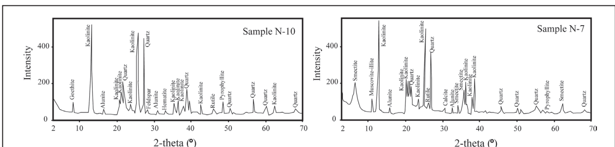
شکل ۵- الگوهای تجزیه XRD برای دو نمونه از پهنه دگرسانی آرژلیک مورد مطالعه.
