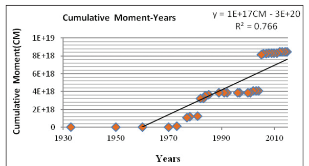
شکل ۳- نرخ گشتاور لرزه‌ای حاصل از زمین‌لرزه‌های دستگاهی برای بخش شمالی منطقه مورد مطالعه (با استفاده از روش رسم نمودار).
