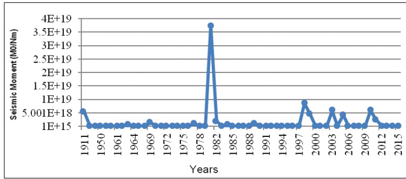
شکل ۷- تغییرات گشتاور لرزه‌ای در طول زمان کاتالوگ لرزه‌ای مورد استفاده (۱۹۱۱-۲۰۱۵). بیشترین مقدار گشتاور لرزه‌ای به ترتیب در سال‌های ۱۹۸۱، ۱۹۹۸، ۲۰۱۰، ۲۰۰۳، ۲۰۱۱، ۱۹۹۹ و ۲۰۰۵ بوده است.
