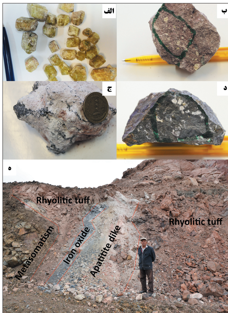
شکل ۳- نمونه‌های آپاتیت مورد مطالعه؛ الف) بلورهای آپاتیت کانسار اسفوردی؛ ب) بلورها و ریزبلورهای آپاتیت کانسار چغارت؛ ج) ریزبلورهای آپاتیت اسفوردی همراه با مگنتیت؛ د) بلورهای آپاتیت در زمینه مگنتیت کانسار چادرملو؛ ه) دایک آپاتیتی نفوذ کرده در توف‌های ریولیتی CVSU در کانسار اسفوردی.
