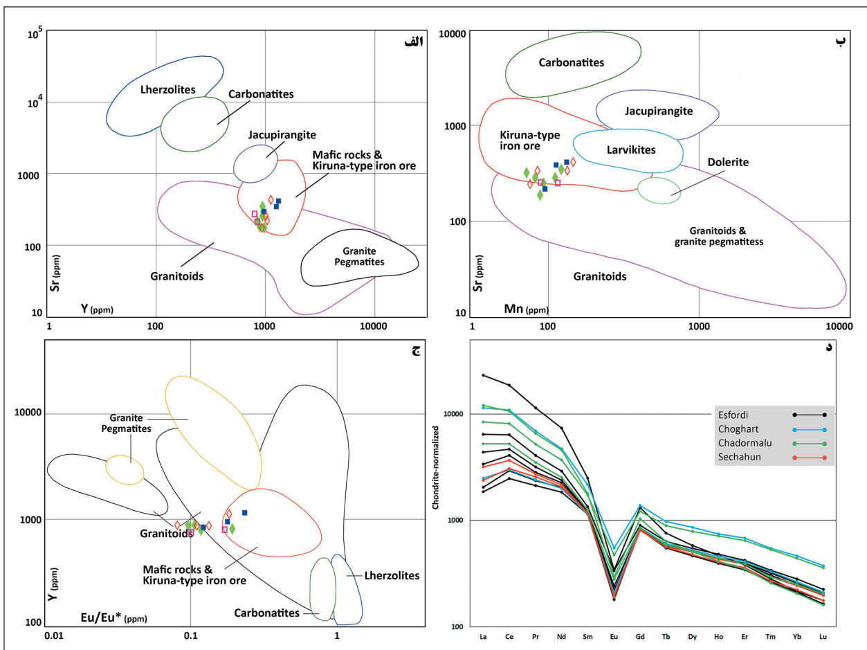
شکل ۵- نمودار ترکیب الف (Sr-Y؛ ب) Sr-Mn؛ ج) Eu/Eu^* بر پایه Belousova et al. (2002). راهنمای نشانه‌های اختصاری از شکل ۴؛ د) نمودار عنکبوتی عناصر خاکی کمیاب بهنجار شده با کندریت (داده‌های کندریت از (Sun and McDonough (1989).
