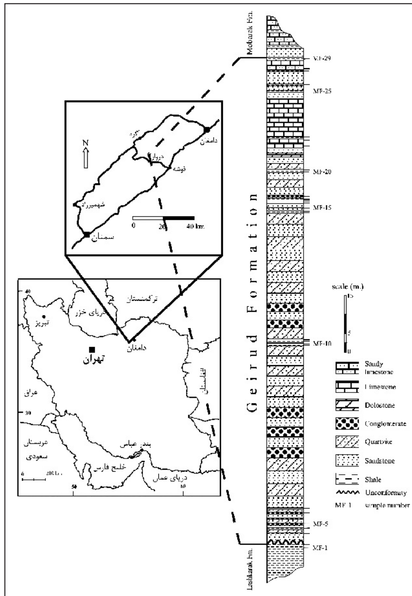
شکل ۱- موقعیت جغرافیایی و ستون چینه‌شناسی سازند جیروود، برش چینه‌شناسی دروار، جنوب باختر دامغان.
