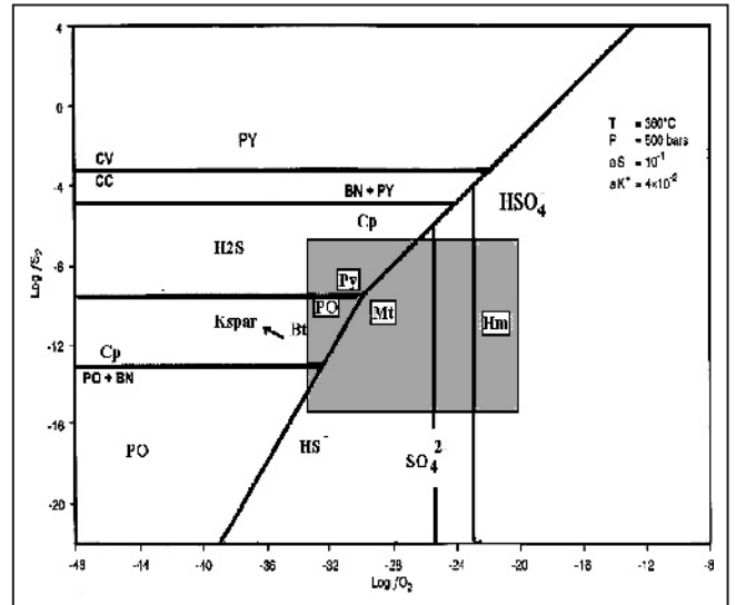
شکل ۹- نمودار با متغیرهای فعالیت f_{S_2} و f_{O_2} ، میدان پایداری کانی‌هایی مثل پیریت، پروتیت، مگنتیت، بورنیت، هماتیت و کانی‌های دگرسانی مثل فلدسپار قلیایی و بیوتیت گرمایی مشخص شده است (برگرفته از Hezarkhani et al., 1999).
