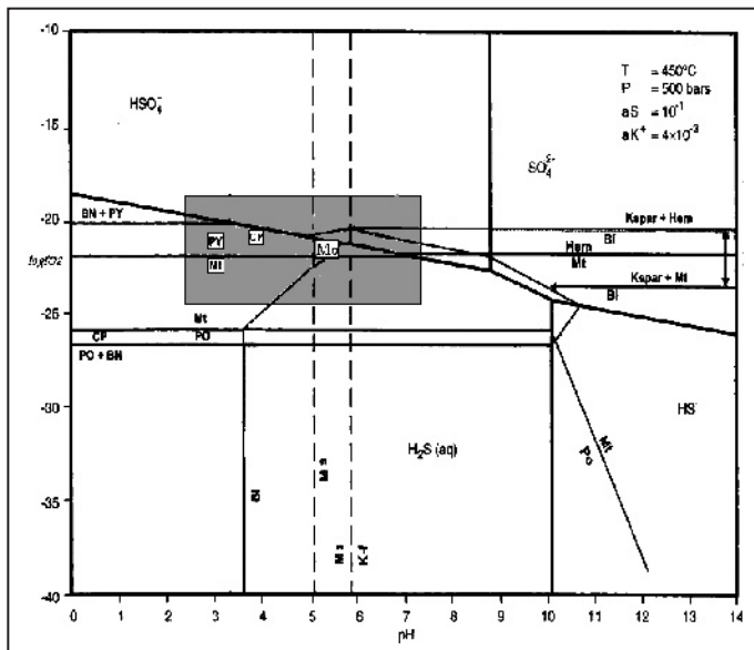
شکل ۷- نمودار هم‌دمای \log fO_2 و pH در دمای ۴۵۰ درجه سانتی‌گراد و فشار ۵۰۰ بار (شرایط برآوردی برای بیشتر کانه‌زایی مولیبدنیت و دگرسانی پتاسیک همراه با آن در سونگون) رسم شده است (بر گرفته از Hezarkhani et al., 1999).
