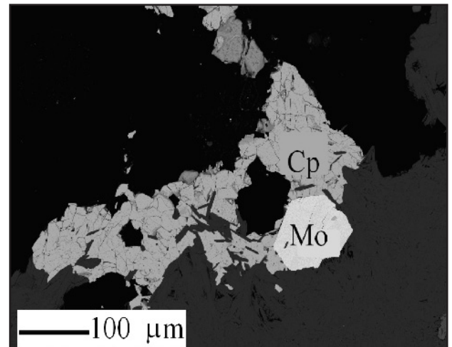
شکل ۶- تصویر BSE از مولیبدنیت هزاگونال و کالکوپیریت در زون پتاسیک.
