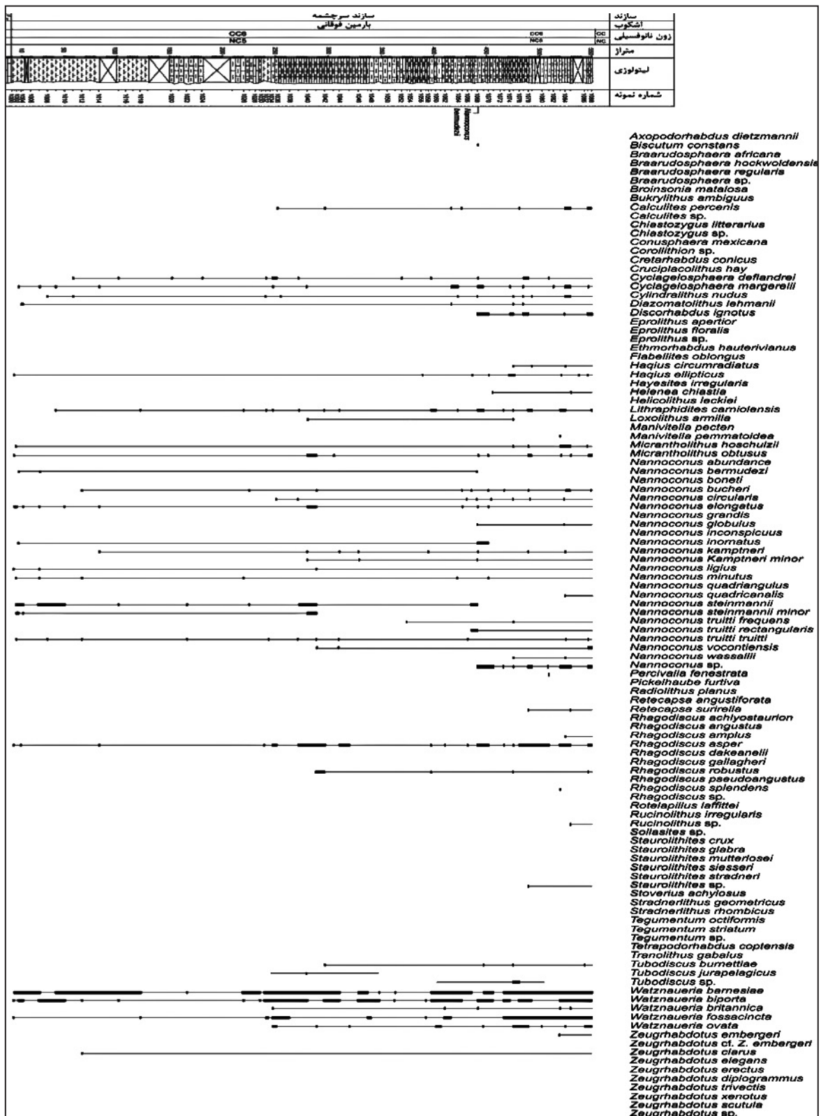
شکل ۵- پراکنده‌گی نانوفسیل‌های آهکی در برش تکل کوه
