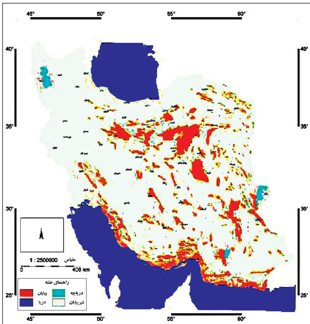
شکل ۷- نقشه بیابان‌های ایران از جنبه عوامل زمین‌شناسی
