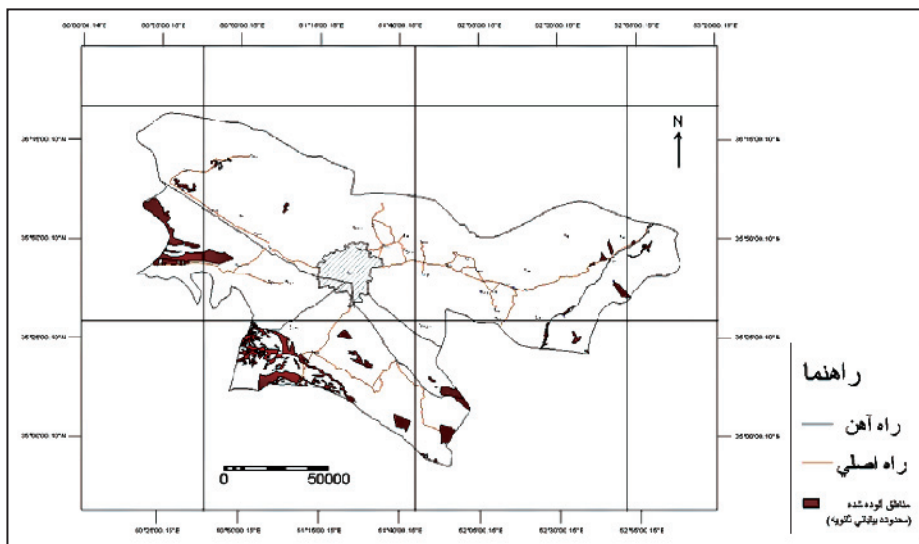
شکل ۳- نقشه سازندهای زمین‌شناسی مؤثر در تشکیل بیابان‌های ثانویه در استان تهران
