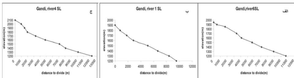
شکل ۳ - نیمرخ‌های گرادیان آبراهه‌های شماره ۱) (ب)، ۴) (ج) و ۶) الف) در محدوده گندی. نیمرخ‌ها در مناطق فعال دارای شکل کوژ به بالا هستند. در شکل ج آشکارا دو بیشینه گرادیان (و در نتیجه SL) در ارتفاعات ۱۸۰۰ و ۱۶۰۰ متر دیده می‌شود. به علت لگاریتمی بودن محور قائم، نیمرخ در مسافت‌های بیش از ۱۰۰۰ متر تدریجاً به خط افقی نزدیک می‌شود. نیمرخ‌ها بر اساس نقشه subenvelope شکل ۲ تهیه شده‌اند. به منظور آشکارتر شدن نیمرخ‌ها، مقیاس افقی (ارتفاعات) نسبت به نقشه پایه اغراق آمیز شده است.
