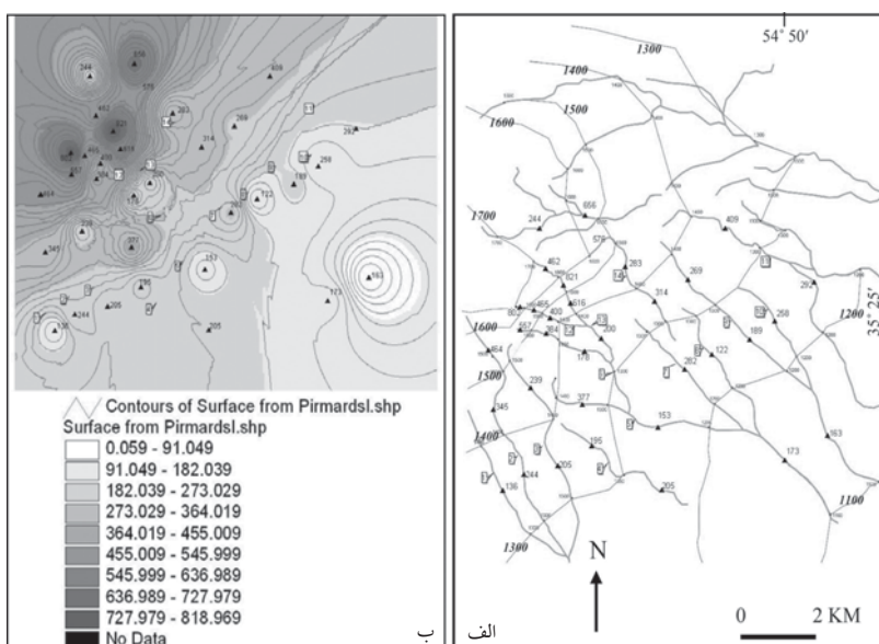
شکل ۶- الف) نقشه subenvelope محدوده پیرمردان. خطوط سبتر پرننگ نشان‌دهنده آبراهه‌ها و خطوط نازک‌تر معرف خطوط تراز وصل‌کننده نقاط هم ارتفاع بستر آبراهه‌ها است. اعداد درشت‌تر مقادیر SL و اعداد درون کادر شماره آبراهه‌های مطالعه شده را نشان می‌دهند. اعداد ایتالیک ارتفاع منحنی‌های subenvelope هستند. نقشه پایه: نقشه توپوگرافی ۱:۵۰۰۰۰ و رنگ عوض، برگ ۶۹۶۰I، سری KV۵۳، سازمان جغرافیایی کشور، ۱۳۵۳. (ب) نقشه منحنی میزان SL بر اساس نقشه ۶-الف در محدوده پیرمردان که مقدار بیشینه SL را در شمال باختر محدوده نشان می‌دهد.
