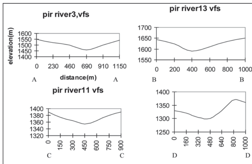
شکل ۱۵ - نیمرخ توپوگرافی تعدادی از آبراهه‌های محدوده پیرمردان که برای محاسبه شاخص Vf تهیه شده است. محل نیمرخ‌ها در شکل ۱۴ مشخص شده است. به منظور آشکارتر شدن نیمرخ‌ها، مقیاس‌های مسافت و ارتفاع اغراق آمیز شده‌اند و با مقیاس شکل ۱۴ تفاوت دارند. مقدار شاخص Vf برای نیمرخ‌های AA تا DD بر اساس شکل ۱۴ محاسبه شده و به ترتیب عبارتند از: ۳/۲؛ ۴/۶؛ ۲/۵؛ ۳/۰۶؛ ۳/۰۶.
