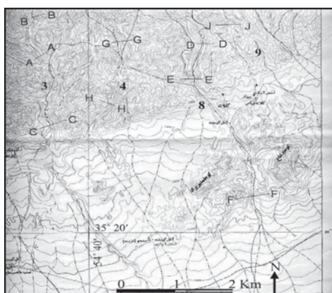
شکل ۱۱- بخشی از نقشه توپوگرافی سدغه (سازمان جغرافیایی کشور، ۱۳۵۳) که در آن محل نیمرخ‌های تعیین شاخص Vf مشخص شده است. اعداد پررنگ بیان گر شماره آبراهه‌های بررسی شده هستند.
