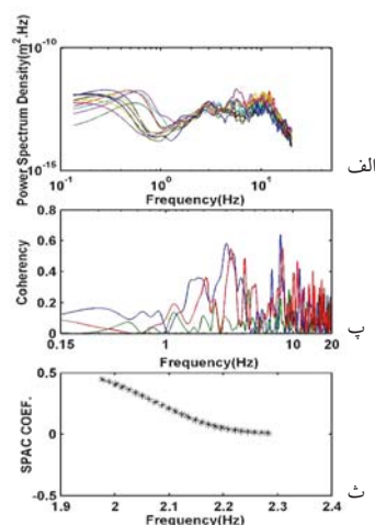
شکل ۵- روند تحلیل داده‌ها به منظور برآورد ضرایب خود همبستگی مکانی و منحنی پاشش در آرایه کوچک به شعاع ۱۴۸ متر (الف) طیف چگالی توان در پنجره‌های زمانی انتخابی (ب) طیف چگالی توان نگاشت‌های میکروترمورها در ۴ ایستگاه آرایه (پ) تابع هم‌دوسی بین جفت ایستگاه‌ها (ت) توابع خود همبستگی مکانی بین جفت ایستگاه‌ها (خطوط رنگی) و تابع میانگین خود همبستگی مکانی (خط سیاه) (ث) تابع میانگین خود همبستگی مکانی در بازه بسامدی که سرعت‌های فاز استخراج شده است (ج) منحنی پاشش به دست آمده در آرایه کوچک
