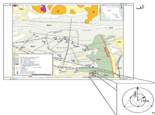
شکل ۳- الف) موقعیت آرایه میکروترمورها مطالعه حاضر (دایره سرخ) به همراه محل نیمرخ‌های درون چاهی مرکز تحقیقات ساختمان و مسکن (مربع آبی) (ب) هندسه و ابعاد آرایه برداشت میکروترمورها
