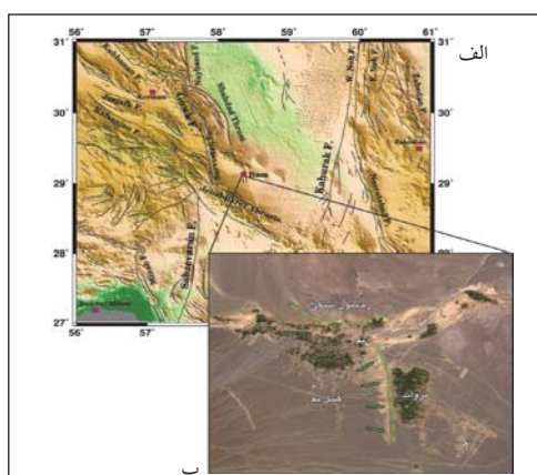
شکل ۱- الف) گسل‌های اصلی پیرامون بم (موقعیت گسل‌ها، طالبیان) (ب) موقعیت شهر بم، رخنمون سنگی آذرین و امتداد جنوبی گسل قدیمی بم بر روی تصویر ماهواره‌ای لندست (LANDSAT)
