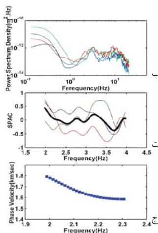
شکل ۵- روند تحلیل داده‌ها به منظور برآورد ضرایب خود همبستگی مکانی و منحنی پاشش در آرایه کوچک به شعاع ۱۴۸ متر (الف) طیف چگالی توان در پنجره‌های زمانی انتخابی (ب) طیف چگالی توان نگاشت‌های میکروترمورها در ۴ ایستگاه آرایه (پ) تابع هم‌دوسی بین جفت ایستگاه‌ها (ت) توابع خود همبستگی مکانی بین جفت ایستگاه‌ها (خطوط رنگی) و تابع میانگین خود همبستگی مکانی (خط سیاه) (ث) تابع میانگین خود همبستگی مکانی در بازه بسامدی که سرعت‌های فاز استخراج شده است (ج) منحنی پاشش به دست آمده در آرایه کوچک
