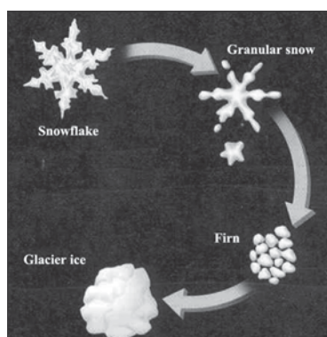
شکل ۱- فرایند تشکیل یخچالی
