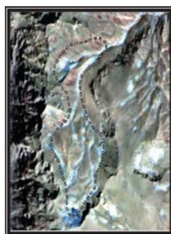
شکل ۱۳- تصویر تلفیق شده Aster و IRS یخچال خرسان و محدوده رقمی شده یخچال
