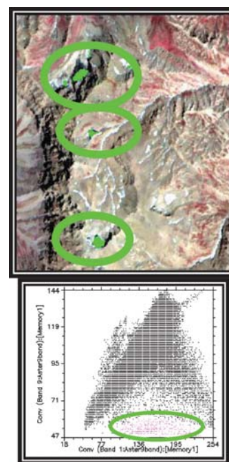
شکل ۶- فضای عارضه مربوط به باندهای ۱ و ۹ سنجنده Aster، منطقه سبز رنگ نشان‌دهنده یخ لخت و یخ سال‌های قبل (Firn) است.
