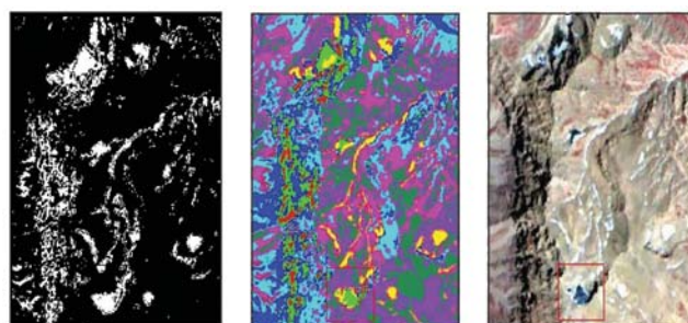
شکل ۴- طبقه‌بندی تصویر Aster سال ۲۰۰۱ یخچال خرسان به روش ISODATA، (الف) تصویر ماهواره‌ای Aster، (ب) تصویر طبقه‌بندی شده با ۱۰ طبقه، (ج) محدوده استخراج شده یخچال
