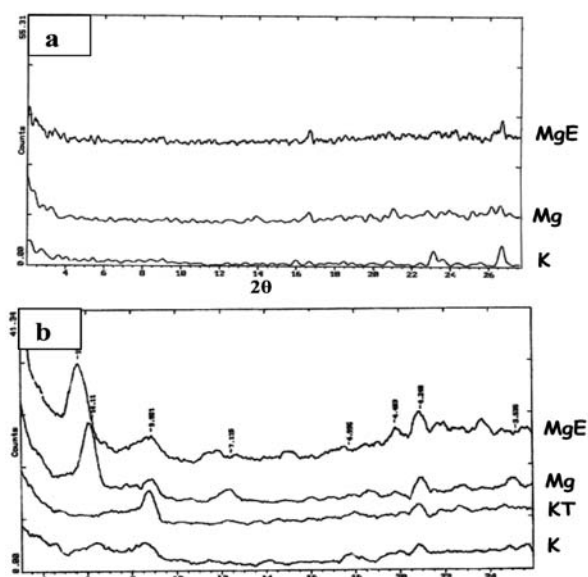
شکل ۷- دو نمونه از نتایج XRD مربوط به مارن های سازند گورپی. (a) نمونه مربوط به مارن پایینی (b) نمونه مربوط به مارن بالایی
