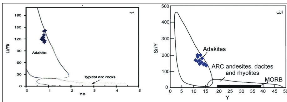
شکل ۸- نمودار Sr/Y در برابر Y و نمودار La/Yb در برابر Yb برای جداسازی سنگ‌های آداکیتی از سنگ‌های عادی مناطق فورانش (Defant and Drummond, 1990). در این نمودارها نمونه‌های مورد مطالعه در جایگاه سنگ‌های آداکیتی قرار می‌گیرند.
