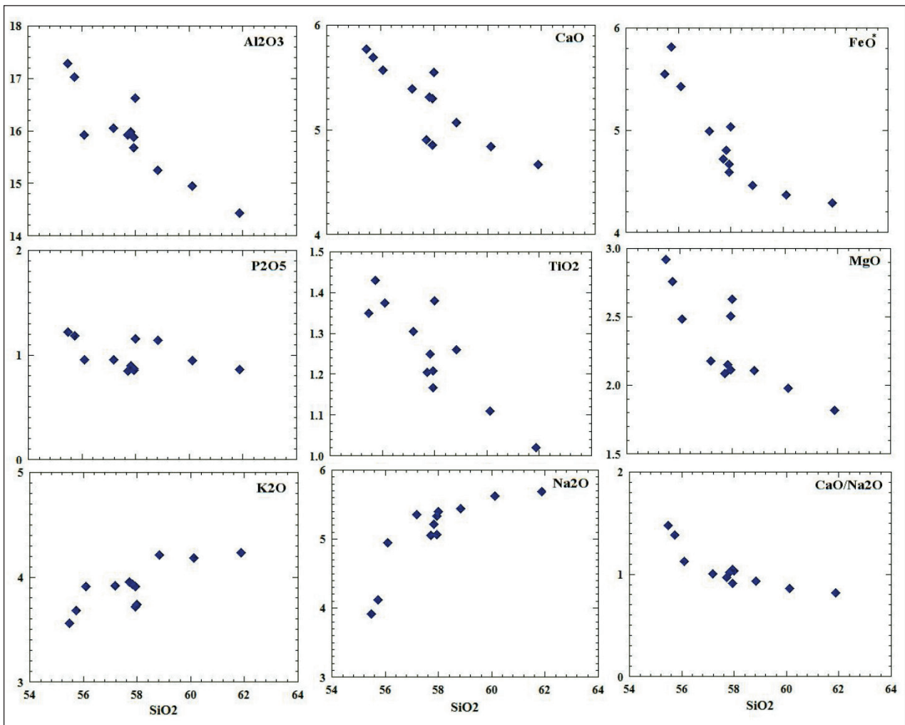
شکل ۵- نمودارهای تغییرات اکسیدهای عناصر اصلی در برابر میزان تغییرات SiO_2 .
