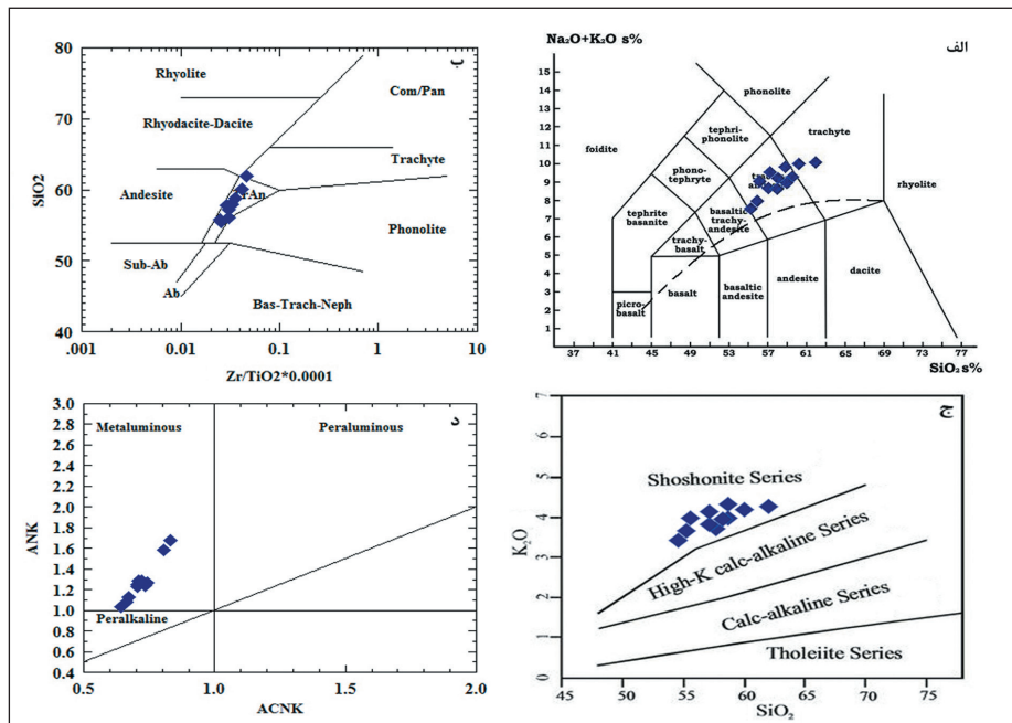
شکل ۶- الف) جایگاه نمونه‌های مورد مطالعه در نمودار SiO 2 در برابر مجموع آلکالی (Le Maitre, 1989). خط معیار جداکننده ساب‌آلکانل و آلکانل از Irvine and Baragar (1971) است؛ ب) موقعیت سنگ‌های مورد مطالعه روی نمودار Zr/TiO 2 در برابر SiO 2 (Winchester and Floyd, 1977)؛ ج) موقعیت نمونه‌های مورد مطالعه در نمودار (Peccerillo and Taylor (1976)؛ د) تعیین درجه اشباع از آلومین بر پایه نمودار (Maniar and Piccoli (1989).
