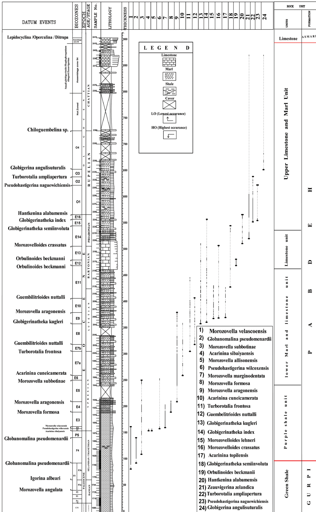
شکل ۶- ستون سنگ‌چینه‌ای و زون‌های زیستی سازند پایده در برش چهارده (پهنه ایده).
