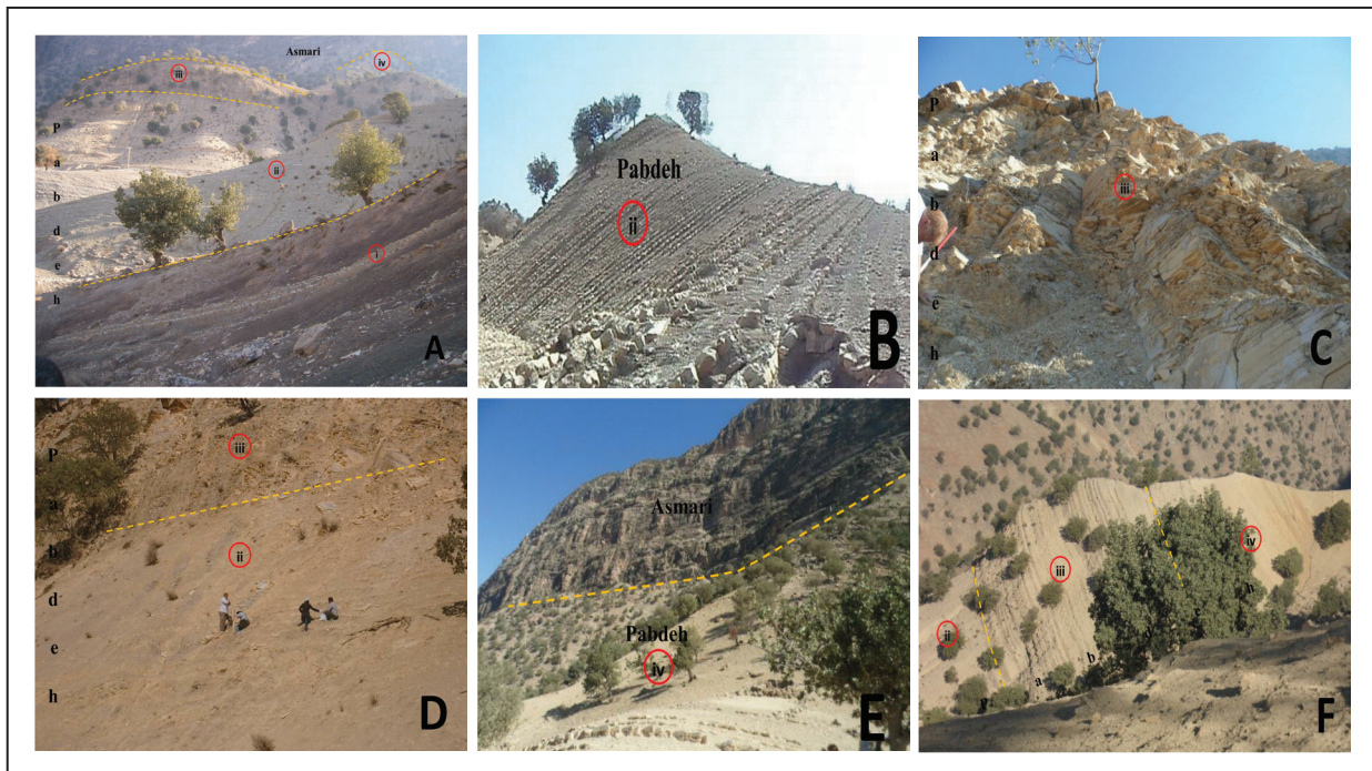
شکل ۴- (A) مرز واحد شیل ارغوانی و واحد مارن و آهک پایینی از سازند پابده در برش چهارده، دید به سوی شمال باختر؛ (B) واحد مارن و آهک پایینی از سازند پابده. دید به سوی شمال باختر؛ (C) واحد آهکی در برش چهارده، دید به سوی شمال باختر؛ (D) مرز واحد مارن و آهک پایینی با واحد آهکی در برش چهارده، دید به سوی شمال باختر؛ (E) مرز واحد مارن و آهک بالایی با سازند آسماری در برش چهارده، دید به سوی شمال باختر؛ (F) مرز مارن و آهک بالایی با واحد آهکی در برش چهارده و مرز واحد آهکی و واحد مارن و آهک پایینی در برش چهارده، دید به سوی شمال باختر (i= شیل ارغوانی و ii= واحد مارن و آهک پایینی، iii= واحد آهکی، iv= واحد مارن و آهک بالایی).
