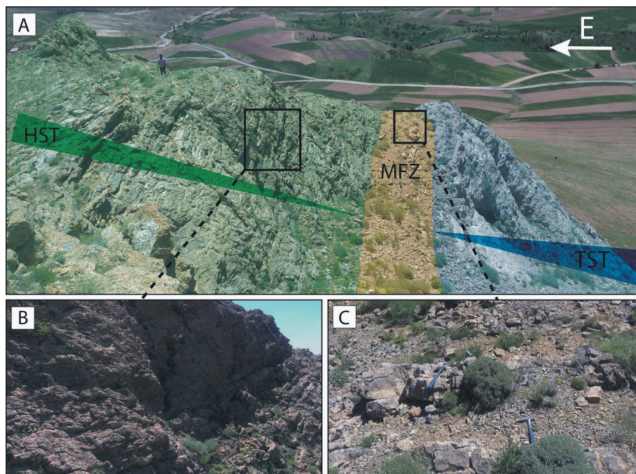
شکل ۱۰- سکانشی رسوبی درجه سوم در بخش‌های سنگ‌آهکی سازند روته در غرب زنجان.
