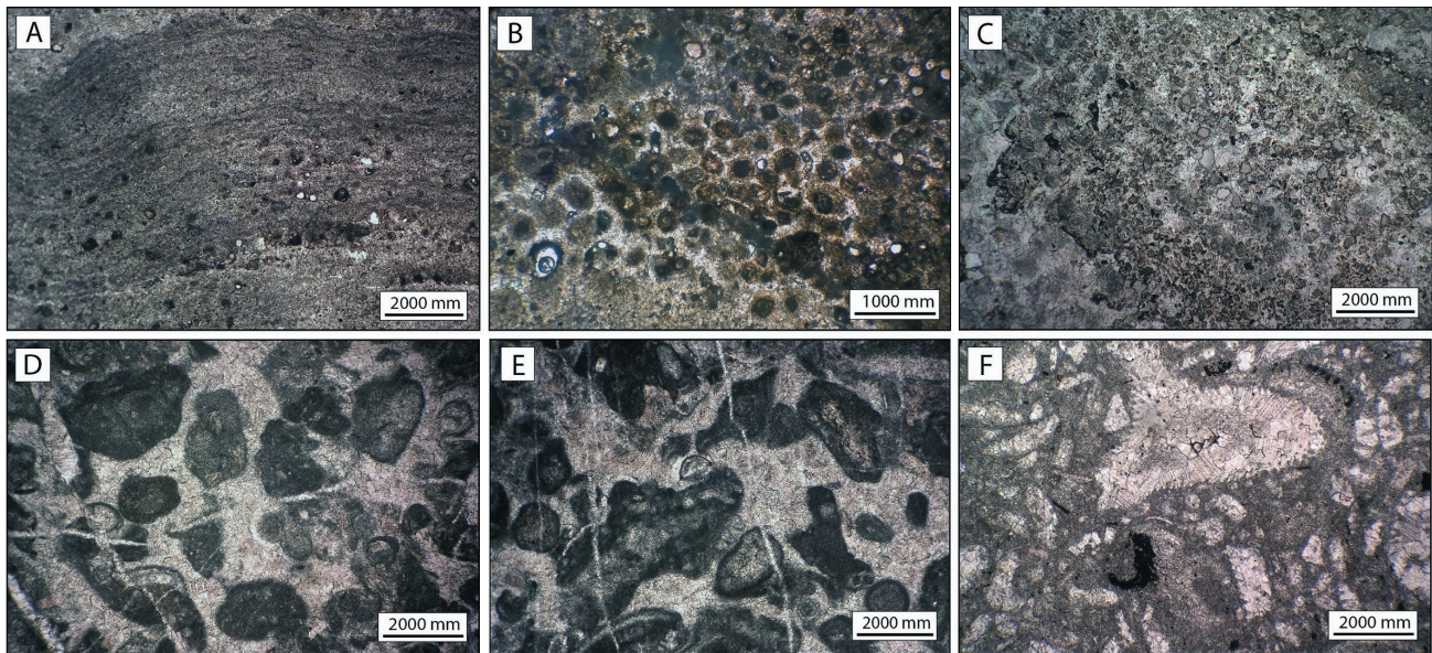
شکل ۶- تصاویر میکروسکوپی از رخساره‌های متعلق به زیر محیط رمپ داخلی سازند روتنه در غرب زنجان؛ (A) رخساره بایندستون حاوی استروماتولیت و پلویید؛ (B) رخساره پکستون تا گریستون حاوی آئید و پلویید؛ (C) فرایند دولومیتی شدن در رخساره پکستون تا گریستون حاوی آئید و پلویید؛ (D و E) رخساره گریستون حاوی پلویید و اینتراکست؛ (F) رخساره وکستون حاوی جلبک سبز.
