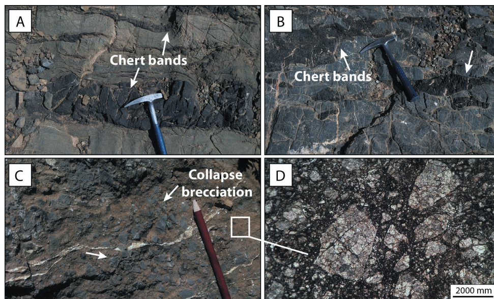
شکل ۱۱- تصاویر صحرایی و میکروسکوپی از بخش‌های بالایی سازند روته در برش مورد مطالعه. (A و B) افق‌های بالایی سازند روته حاوی نوارهای چرت موازی با لایه‌بندی؛ (C و D) برشی شدن سنگ‌آهک‌های دولومیتی که احتمالاً در نتیجه انحلال تحت‌الجوی تشکیل شده است.
