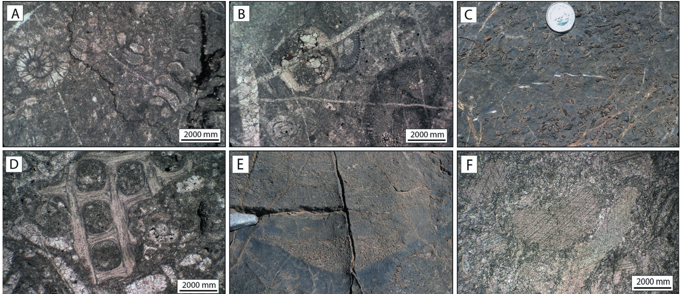
شکل ۷- تصاویر صحرایی و میکروسکوپی از رخساره‌های متعلق به زیرمحیط‌های رمپ داخلی و میانی سازند روته در غرب زنجان (A) رخساره و کستون حاوی فرامینیفرهای بنتیک کوچک؛ (B) رخساره و کستون حاوی جلبک و فرامینیفرهای بنتیک کوچک؛ C و D) رخساره و کستون حاوی جلبک سبز، براکیوپود و خارپوست؛ E و F) رخساره و کستون تا پکستون حاوی خارپوست.
