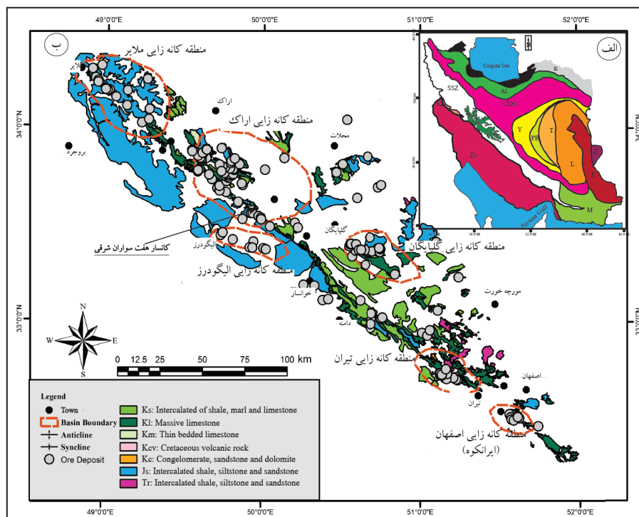
شکل ۱- الف) نقشه زون‌های ساختاری ایران و موقعیت کمربند ملایر- اصفهان درون زون ساختاری سنندج- سیرجان (SSZ) (منطقه سبز رنگ) (آقائباتی، ۱۳۸۳)؛ ب) کمربند فلززایی روی-سرب رسوبی و مناطق شش‌گانه در کمربند فلززایی روی-سرب ملایر- اصفهان (Momenzadeh, 1976). Al: البرز؛ CIGS: زون ساختاری و زمین‌شناسی ایران مرکزی؛ E: محدوده شرقی ایران؛ K: کپه‌داغ؛ KR: زیر زون رادیولاریتی کرمانشاه؛ L: بلوک لوت؛ M: زون مکران؛ O: کمربند اوفیولیتی؛ PB: بلوک پشت‌بادام؛ SSZ: زون ساختاری سنندج- سیرجان؛ T: بلوک طبرستان؛ Y: بلوک یزد؛ Z: محدوده زابل؛ Za: محدوده زاگرس.
