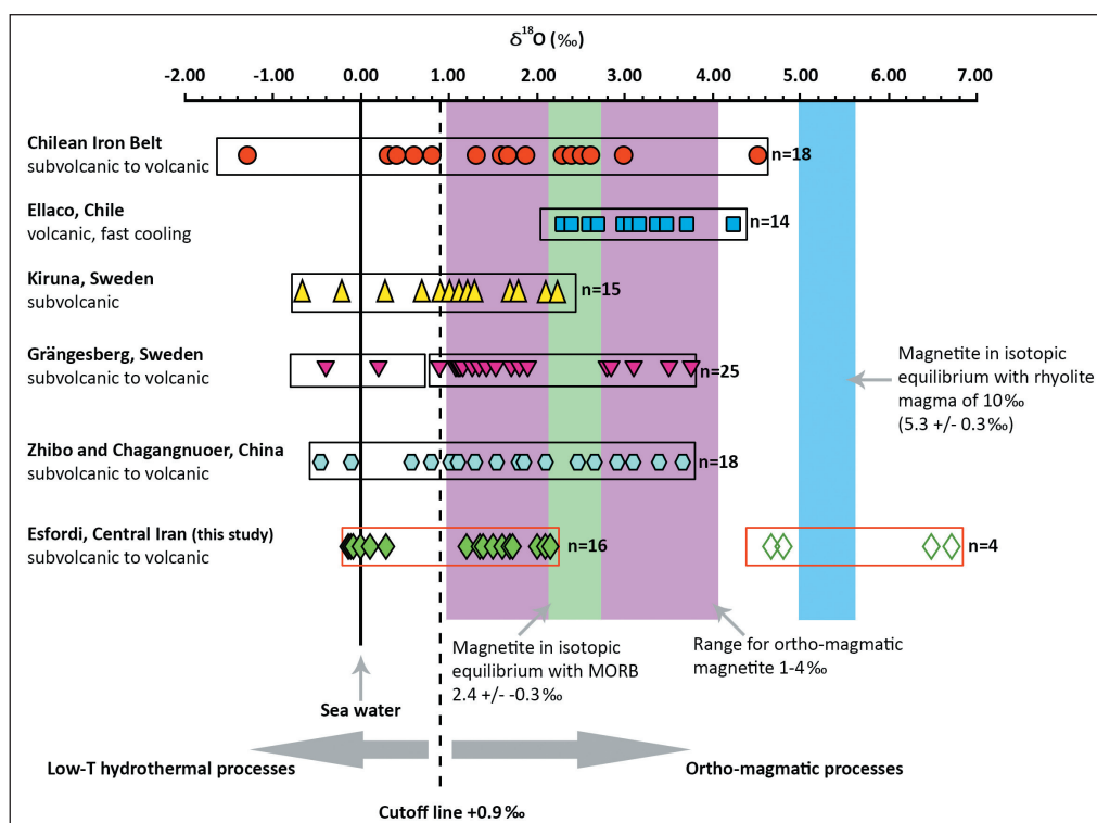
شکل ۳- مقادیر \delta^{18}\text{O} برای مگنتیت‌های کانسارهای چغارت، چادرملو، سه‌چاهون و اسفوردی. داده‌های کانسارهای کمر بند آهن و کانسار ال‌لاکو در شیلی (Nystrom et al., 2008)، کانسارهای کایرونا (Jonsson et al., 2011) و گرانگبرگ (Weis, 2013) در سوئد و کانسارهای ژیبو و چاگانگوئر در چین (Zhang et al., 2014).
