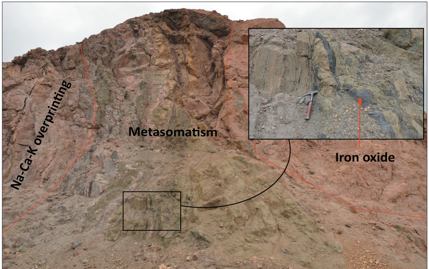
شکل ۲- متاسوماتیسم آلکالن رخ داده در سنگ میزبان کانه‌زایی.
