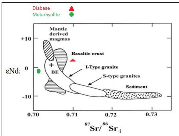
شکل ۹- نمایش تغییرات میزان ^{87}\text{Sr}/^{86}\text{Sr} اولیه در مقابل \epsilon\text{Nd}_i برای متاریولیت و دیاباز دامن قر جهت تعیین منشأ سنگ (Keay et al., 1997).
