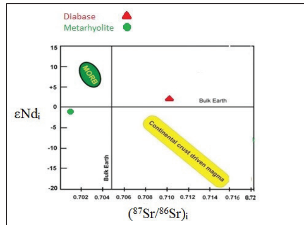
شکل ۷- نمودار موقعیت مکانی متاریولیت و دیاباز دامن قر بر اساس مقادیر نسبت ( ^{87}\text{Sr}/^{86}\text{Sr} ) اولیه در مقابل \epsilon\text{Nd} . منابع برای پوسته بالایی (Taylor and McLennan, 1985) و (Rollinson, 1993; Sun and Mc donough, 1989) MORB
