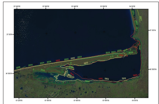
شکل ۶- مقایسه خطوط ساحلی در سال‌های مختلف.
