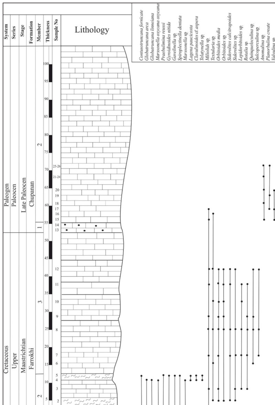
شکل ۷- ستون چینه‌شناسی و گسترش چینه‌شناسی روزن‌بران در برش زالوبند.
