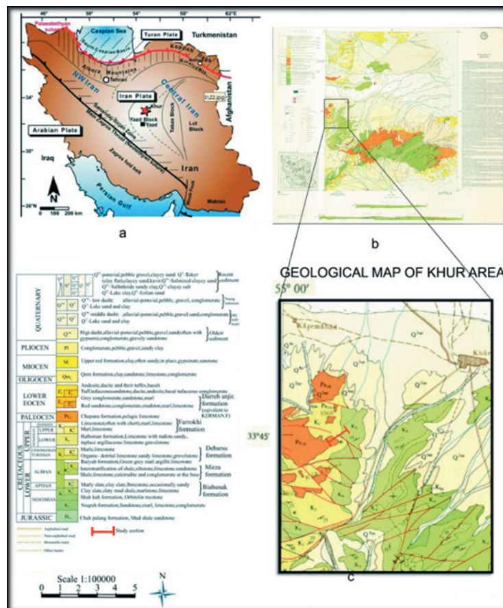
شکل ۳- موقعیت زمین‌شناسی برش هونو: (a) موقعیت برش مورد مطالعه در بلوک یزد (Wilmsen et al., 2012)؛ (b و c) نقشه ۱:۱۰۰۰۰۰ خور (سازمان زمین‌شناسی و اکتشاف معدنی کشور).
