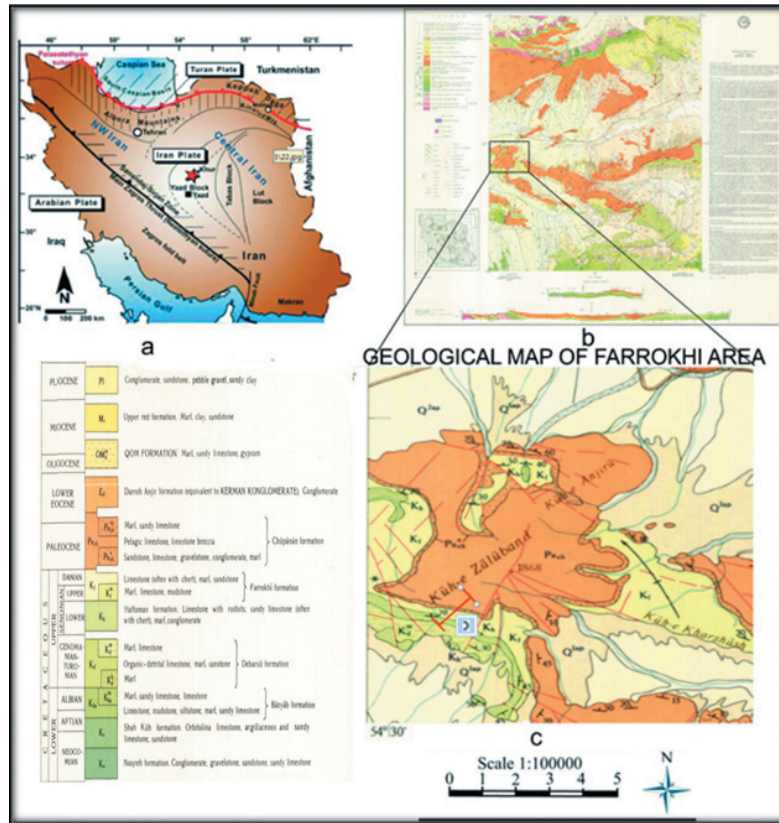
شکل ۲- موقعیت زمین‌شناسی برش زالویند: (a) موقعیت برش مورد مطالعه در بلوک یزد (Wilmsen et al., 2012)؛ (b و c) نقشه ۱:۱۰۰۰۰۰ فرخی (سازمان زمین‌شناسی و اکتشاف معدنی کشور).
