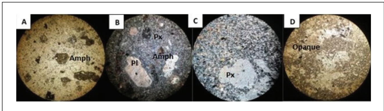
شکل ۳- (A) بلورهای آمفیبول با رخ منشوری (PPL)؛ (B) بلورهای آمفیبول، پیروکسن و پلاژیوکلازهای دگرسان شده با بافت غربالی و خوردگی خلیجی (XPL)؛ (C) بلورهای پیروکسن (XPL)؛ (D) حضور کانی‌های کدر به صورت اولیه و ثانویه (PPL) در سنگ‌های داسیتی- شعاع میدان دید ۲۰/۸ میلی متر.
