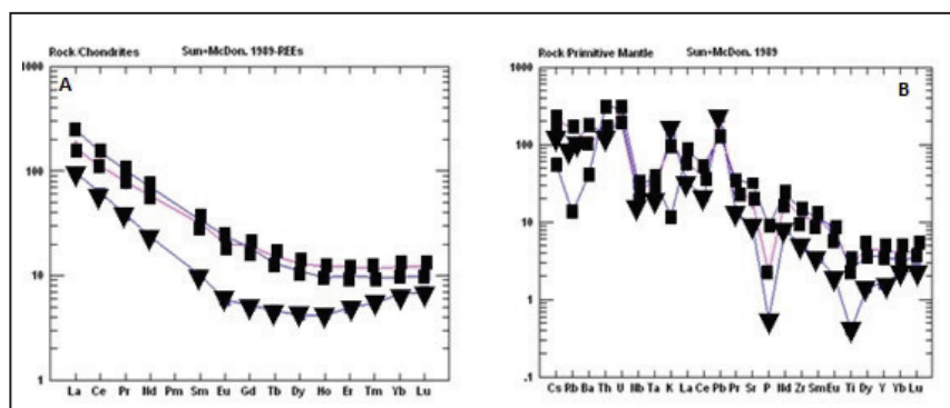
شکل ۷- (A) نمودار عناصر نادر خاکی؛ (B) نمودارهای چند عنصری سه نمونه منتخب از واحدهای مورد مطالعه (Sun and McDonough, 1989).
