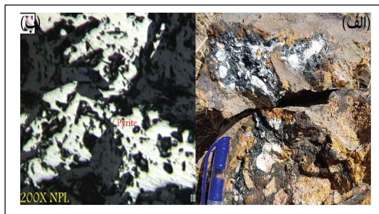
شکل ۱۱- رگچه‌های کوارتز سولفیددار مربوط به مرحله دوم و فاز سوم کانه‌زایی به‌صورت رگچه‌های سیلیسی-سولفیدی و برشی بافت توده‌ای در سولفیدها.
