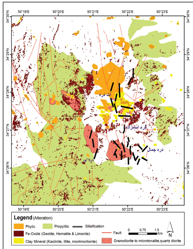
شکل ۷ - تفکیک انواع دگرسانی‌ها و ارتباط آن با توده‌های نیمه‌عمیق و گسل‌ها در محدوده معدنی ۱/۲۵۰۰ زواریان با استفاده از تصاویر ماهواره‌ای، برداشت‌های صحرایی و مطالعات صورت گرفته در محدوده مورد مطالعه.
