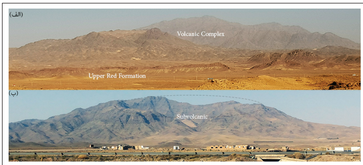
شکل ۳- نمائی از محدوده مورد مطالعه: (الف) موقعیت واحدهای رسوبی الگومیوسن نسبت به فعالیت‌های آتشفشانی که ارتفاعات را تشکیل می‌دهند (دید به سمت شمال غرب)، (ب) نمائی نزدیک‌تر از مخروط آتشفشانی میزبان کانه‌زائی زواریان دید به سمت شمال.
