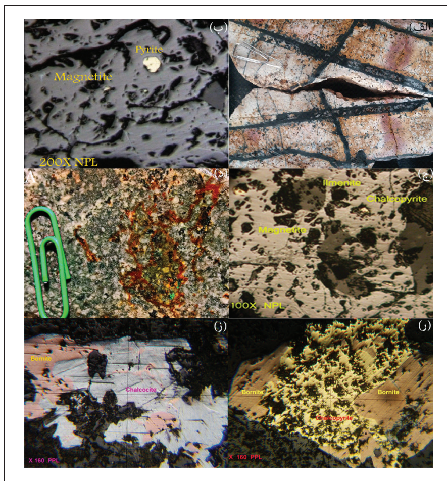
شکل ۱۰- نمایی از فازهای دگرسانی و مراحل کانه‌زایی، الف) رگه- رگچه‌های سیلیسی مگنتیتی مرحله دوم و فاز اول کانه‌زایی در نمونه دستی؛ ب-ج) ادخال‌های کوچک پیریت و کالکوپیریت در رگه‌های مگنتیتی- ایلمنیتی فاز اول از مرحله دوم کانه‌زایی؛ د) نمونه دستی از رگچه‌های کوارتز تورمالین و مس‌دار مرحله دوم و فاز دوم کانه‌زایی؛ ر-ز) دانه‌های درشت کالکوپیریت، بورنیت (ر) و بورنیت- کالکوسیت (ز) به صورت هم‌رشد و محلول جامد را در محدوده آت دره نشان می‌دهند (عکس ر- ز برگرفته از روزبه کارگر و موحدی، ۱۳۸۹).
