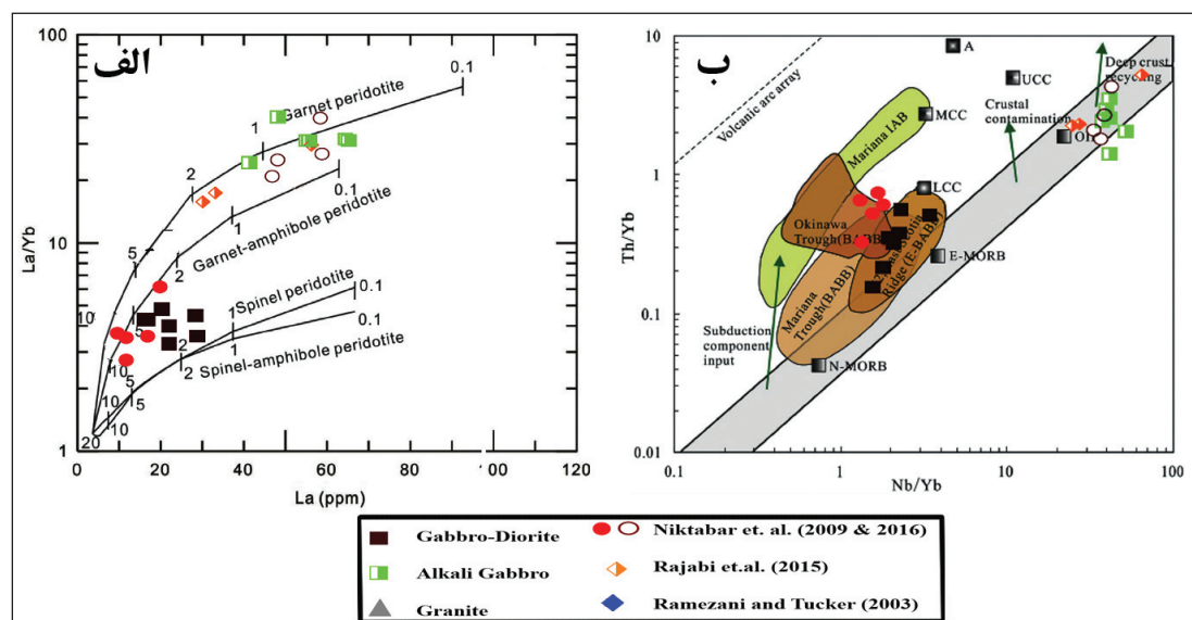
شکل ۱۳ - موقعیت نمونه‌های منطقه زیرگان در: الف) مدل سازی ذوب بخشی منابع مختلف گوشته در نمودار La/Yb در مقابل La (به نقل از Jiang et al. 2018). ب) نمودار Th/Yb-Nb/Yb (Pearce, 1982) اصلاح شده توسط (Liu et al., 2018).
