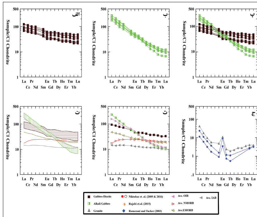
شکل ۱۰- الگوی عناصر کمیاب خاکی بهنجار شده به کندریت (Sun and McDonough, 1989) (الف) گابرو-دیوریت. (ب) آلکالی گابرو. (پ) گابرو-دیوریت و آلکالی گابرو. (ت) گابرو-دیوریت و آلکالی گابرو در مقایسه با میانگین، NMORB، OIB و EMORB (داده‌ها از Niu & O'Hara, 2003). (ث) میانگین گابرو-دیوریت و آلکالی گابرو در مقایسه با میانگین. (ج) نمونه گرانیت زیریگان.
