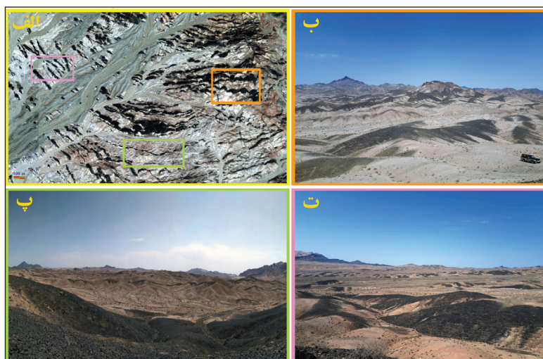
شکل ۳- الف) تصویر ماهواره‌ای از چرخش چپ گرد دایک‌ها و تشکیل ساختار چشمی شکل (طول تصویر ۲۴۶۰ متر). ب، پ و ت) نفوذ دایک‌ها در گرانیت زیرین.
