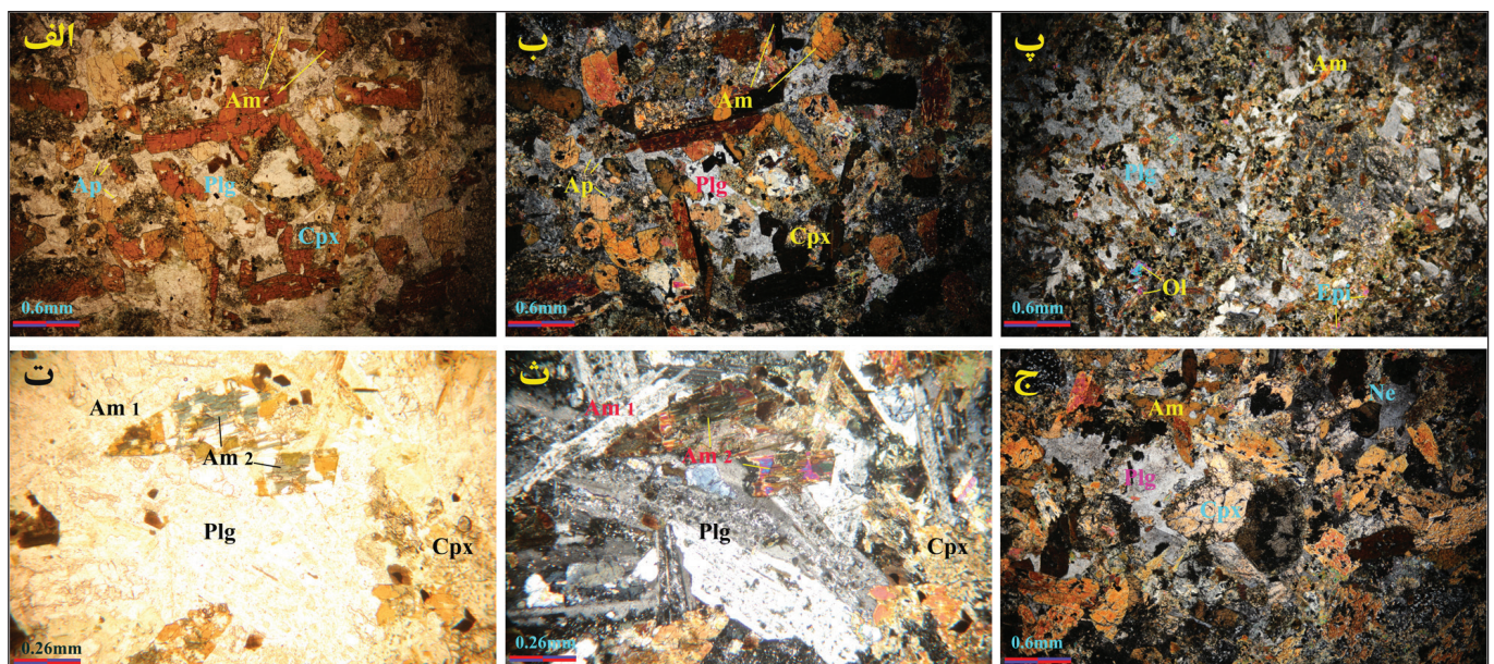
شکل ۶- تصاویر میکروسکوپی دایک‌های آلکالی گابرو: الف) آمفیبول‌های قهوه‌ای از نوع کرسوتیت و کلینوپروکسن (PPL). ب) همان در XPL. پ) بافت افیتیک و بلور الیوین (XPL). ت) تبدیل کرسوتیت به آمفیبول‌های سبز در مراحل بعدی (PPL). ث) همان در XPL. ج) بلور نفلین (XPL).
