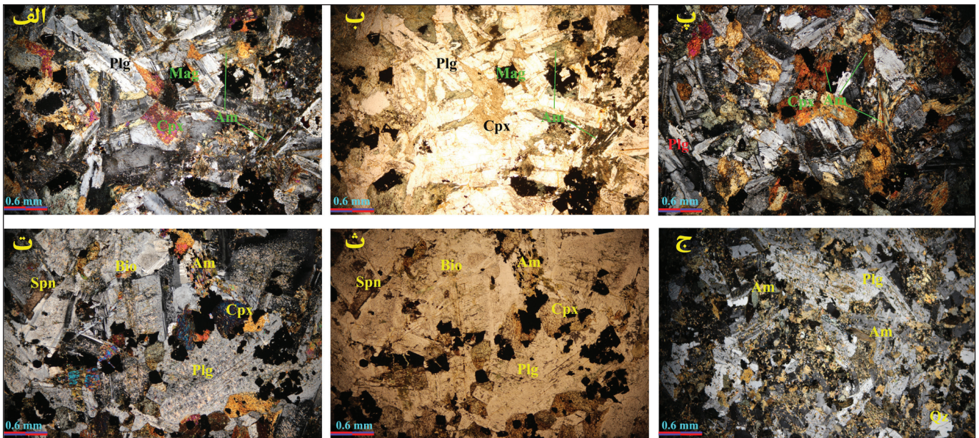
شکل ۵- تصاویر میکروسکوپی دایک‌های گابرو-دیوریتی: الف) بافت اینترگرانولار در مرکز دایک‌های ضخیم (XPL). ب) همان در PPL. پ) کلینوپروکسن‌های در حال تبدیل به آمفیبول سبز (XPL). ت) بافت اینترگرانولار تا ساب افیتیک و پلاژیوکلازهای سوسوریتی (XPL). ث) همان در PPL. ج) حضور کانی کوآرتز در انواع تفریق یافته‌تر کوآرتزدیوریتی (XPL).
