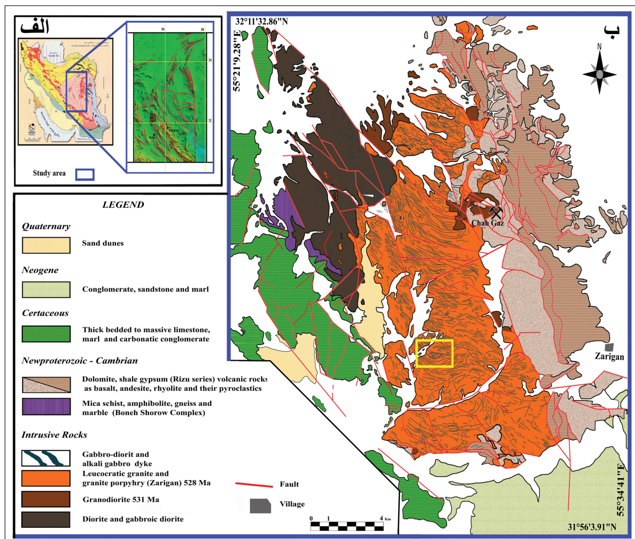
شکل ۱-الف) موقعیت منطقه مورد مطالعه در پهنه‌های زمین‌ساختاری و رسوبی ایران (آقاباتی، ۱۳۸۳). ب) نقشه زمین‌شناسی ۱:۲۰۰۰۰ گرانیته زیرگان و فوج دایک‌های آن (کادر زرد رنگ موقعیت شکل ۳-الف).
