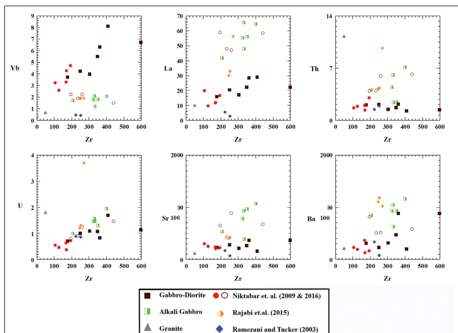
شکل ۹ - تغییرات عناصر کمیاب در برابر Zr.
