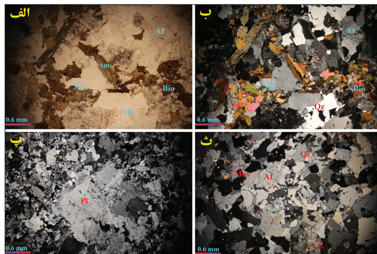
شکل ۲- (الف) نمای میکروسکوپی گرانودیوریت و بلورهای آمفیبول و بیوتیت (PPL). (ب) همان در XPL. (پ) بافت پورفیریوئیدی و هم‌رشدی میرمیکیتی در گرانیت زیرگان (XPL). (ت) بافت گرافیکی در گرانیت زیرگان (XPL).
