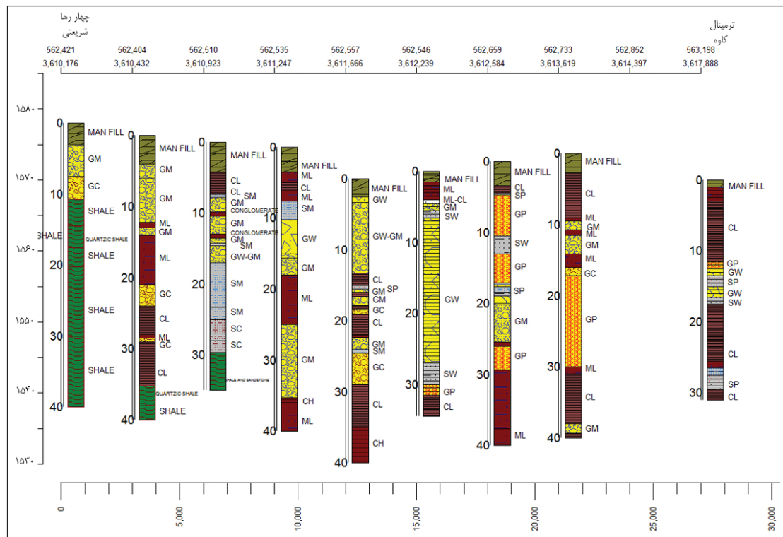
شکل ۵- مقطع زمین شناسی شماره ۱ جنوبی- شمالی (چهار راه شریعتی- ترمینال کاوه).
