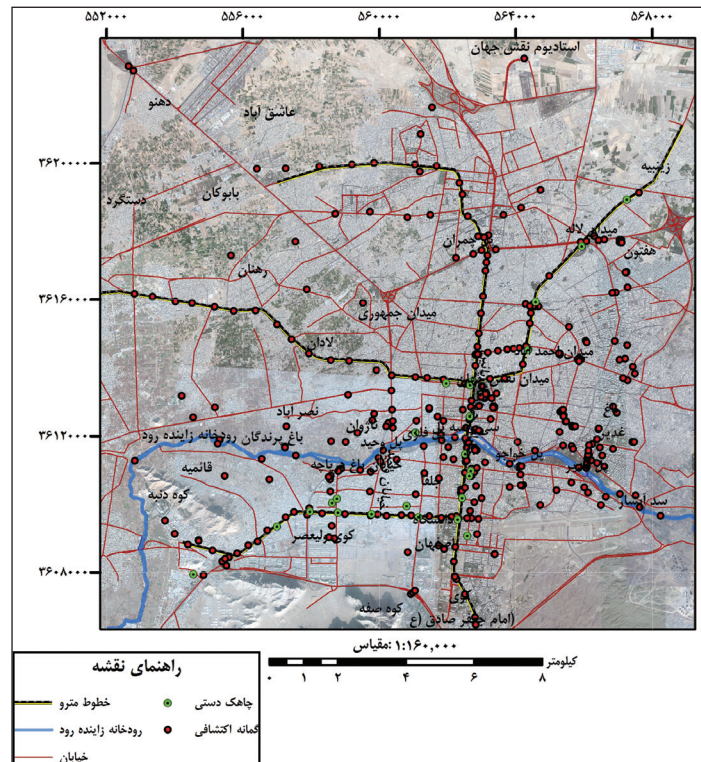
شکل ۳- موقعیت گمانه ها و چاهک‌های اکتشافی بر روی نقشه شهر اصفهان.
