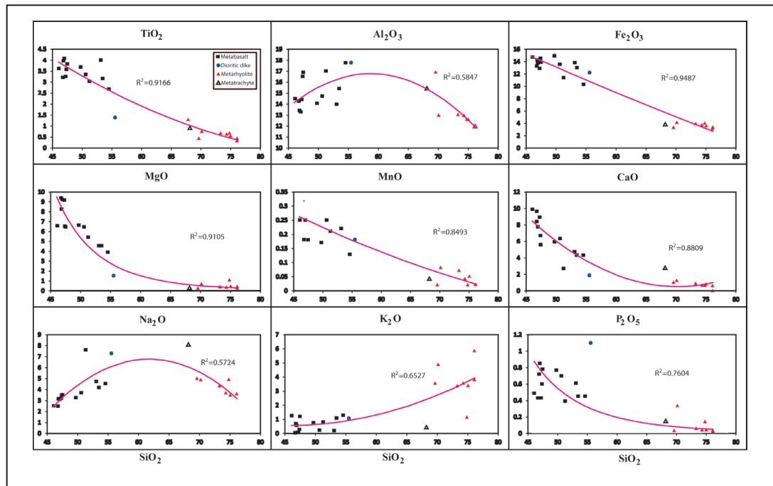
شکل ۹- نمودار تغییرات اکسیدها نسبت به \text{SiO}_2 .
