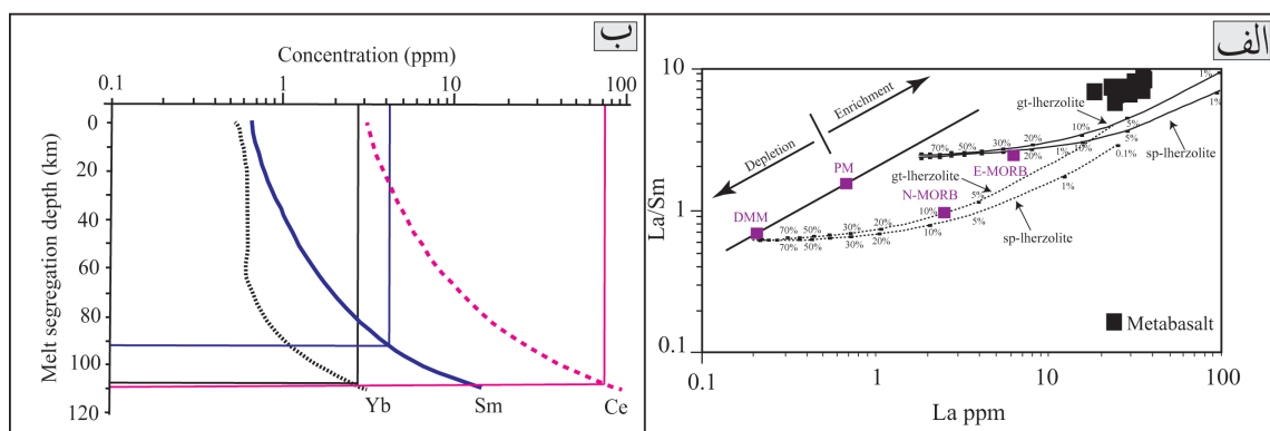
شکل ۱۵- الف) نمودار La/Sm در برابر La ، به منظور محاسبه میزان ذوب بخشی (Aldanmaz et al., 2000)؛ ب) تعیین ژرفای منشأگیری ماگما بر پایه میانگین تمرکز عناصر Sm، Yb و Ce (Ellam, 1992)
