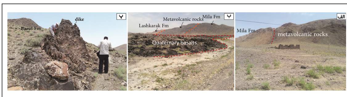
شکل ۴-الف) کنتاکت سازند میلا با سنگ‌های متاولکانیکی اسیدی در اطراف روستای خرز (دید به سمت شمال خاور). ب) نمایی کلی از سازندهای میلا، لشگرک و سنگ‌های متاولکانیکی با ترکیب بازیک (دید به سمت شمال باختر). پ) برونزد دایک نفوذ کرده درون سازند باروت (دید به سمت شمال باختر).
