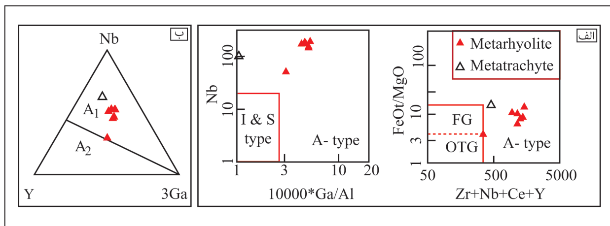
شکل ۱۳- تعیین نوع سنگ‌های مورد بررسی با استفاده از نمودارهای پیشنهادی (Whalen et al. (1987؛ (ب) تشخیص تیپ نمونه‌های مورد مطالعه از طریق نمودارهای پیشنهادی (Eby (1992)
