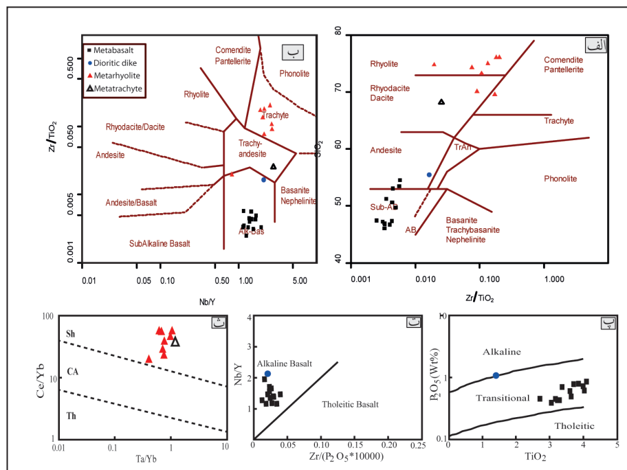
شکل ۸- نمودارهای طبقه‌بندی و تعیین سری ماگمایی، الف) Zr/TiO_2 در برابر SiO_2 ؛ ب) نمودار طبقه‌بندی Zr/TiO_2 در برابر Nb/Y (Winchester and Floyd, 1977)؛ پ) نمودار TiO_2 در برابر P_2O_5 (Floyd and Winchester, 1975)؛ ت) نمودار Nb/Y در برابر (Zr/P_2O_5) \times 10^{-4} (Winchester and Floyd, 1976)؛ ث) نمودار Ce/Yb در برابر Ta/Yb (Pearce, 1983).
