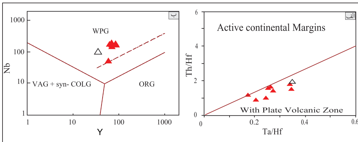
شکل ۱۴- موقعیت نمونه‌های مورد مطالعه در نمودارهای زمین‌ساختی ارائه شده توسط: الف) (Schandle and Gorton (2002)؛ ب) (Pearce et al. (1984)
