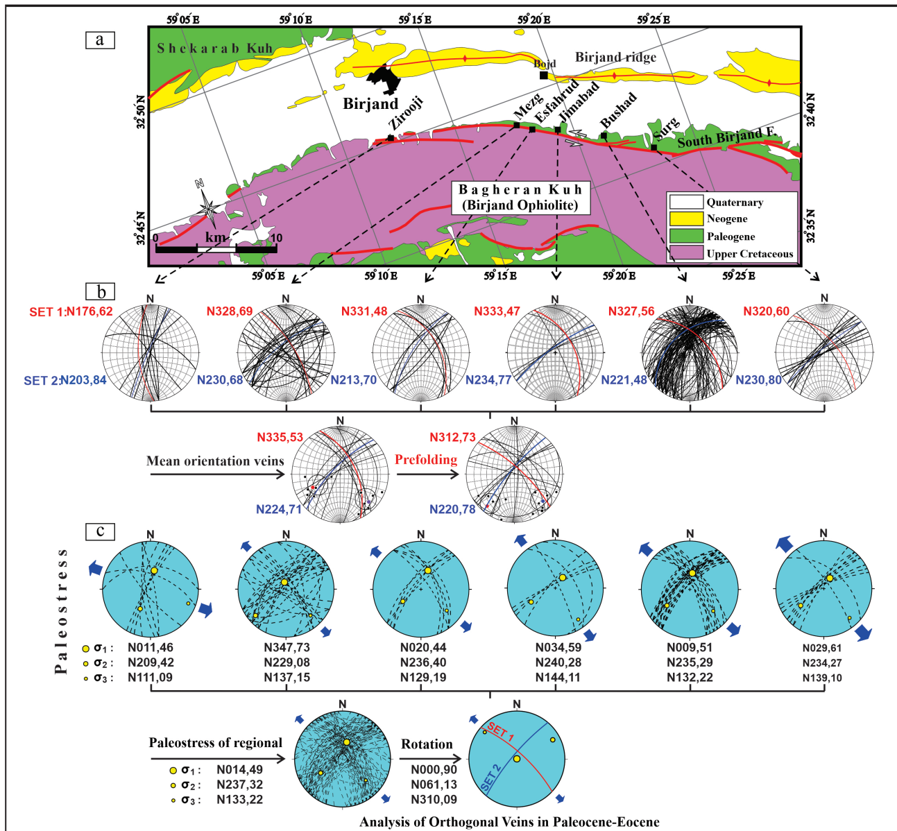
شکل ۴-ا نقشه زمین‌شناسی ساده شده منطقه بیرجند با اصلاحاتی از نقشه زمین‌شناسی ۱:۲۵۰۰۰۰ بیرجند (Vahdati Daneshmand et al., 1991) به همراه موقعیت ایستگاه‌های برداشت داده‌های ساختاری؛ ب) استریوپلات‌ها جهت‌گیری میانگین دسته رگه‌های راست‌گوشه را در رخساره فلیشی جنوب بیرجند برای ۶ ایستگاه نشان می‌دهد؛ ج) بازسازی تنش دیرین با استفاده از رگه‌های راست‌گوشه در این مطالعه.
