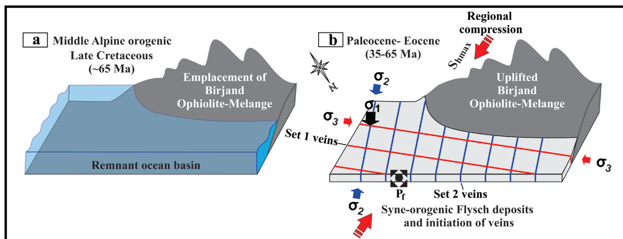
شکل ۶- الگوی تکامل زمین‌ساختی حوضه فلیشی جنوب بیرجند. الف) جایگیری افیولیت ملائز بیرجند در کرتاسه پسین؛ ب) رسوب‌گذاری رخساره فلیشی همزمان با کوهزایی و ایجاد رگه‌های راست گوشه در پالنوسن- انوسن.
