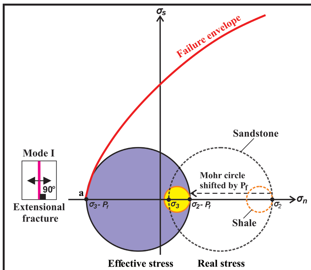
شکل ۵- نمودار گسیختگی مور-گریفیث-کولمب (Bons et al., 2012). فشار سیال ( P_f ) دایره مور را به سمت پوش گسیختگی جابه‌جا می‌کند و تنش موثر ( \sigma_n - P_f ) باعث شکست سنگ می‌شود. شکستگی‌های کششی (حالت I)، زمانی ایجاد می‌گردد که دایره مور پوش گسیختگی را در نقطه a لمس کند. ماسه‌سنگ نسبت به شیل تنش تفاضلی بالاتری دارد در نتیجه در توالی فلیشی، شکستگی کششی اغلب در ماسه‌سنگ ایجاد می‌شود.
