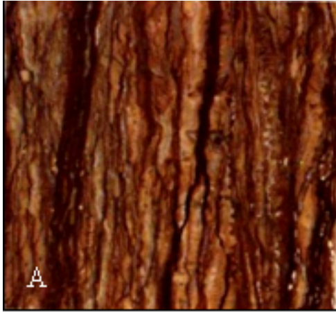
شکل ۴- A) تراورتن گردویی آذر شهر (B) مقطع میکروسکوپی تراورتن گردویی آذر شهر (PPL)
